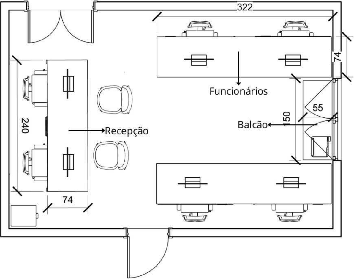
Planta Baixa MEDIDAS: cm
