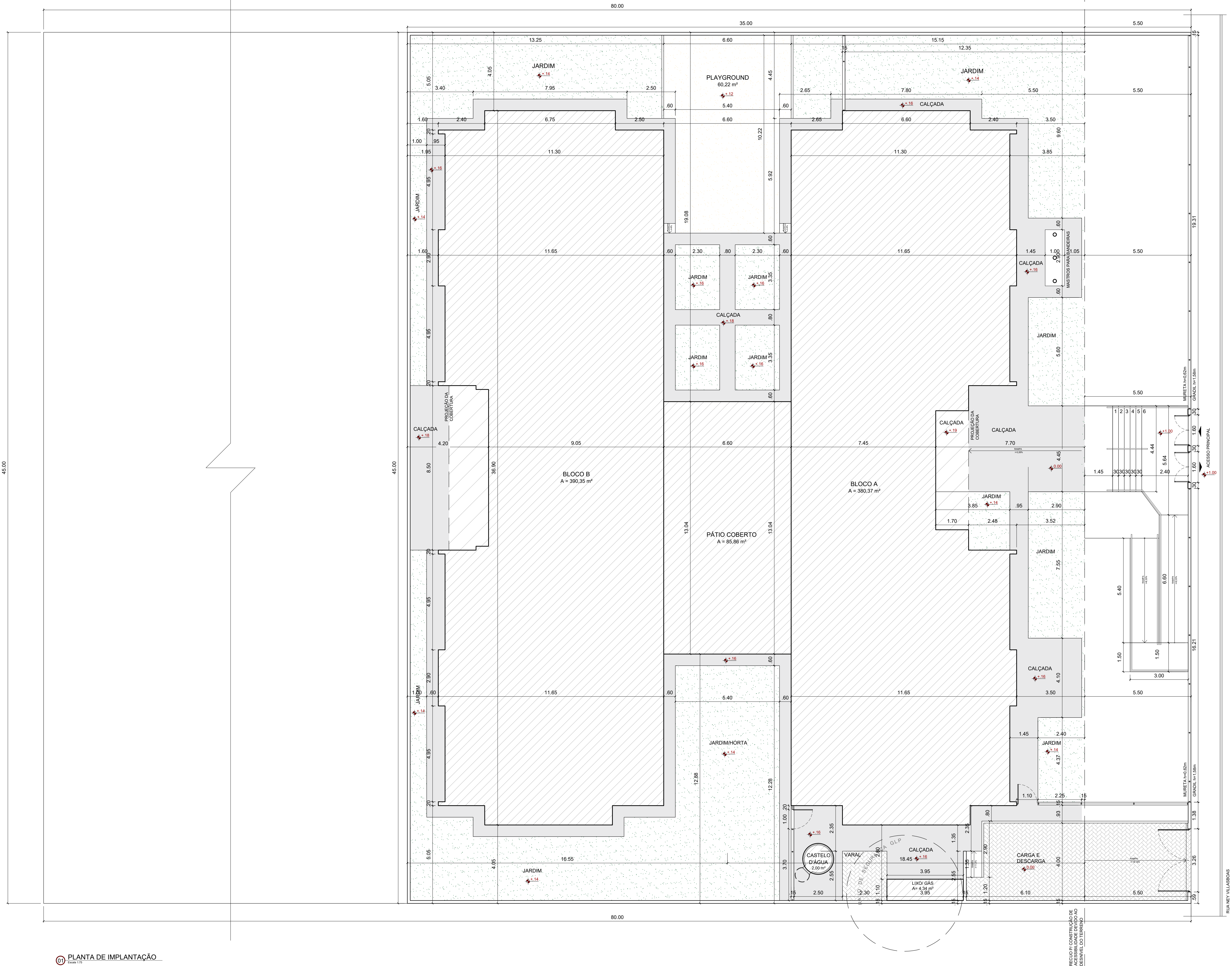
01 PLANTA DE IMPLANTAÇÃO
