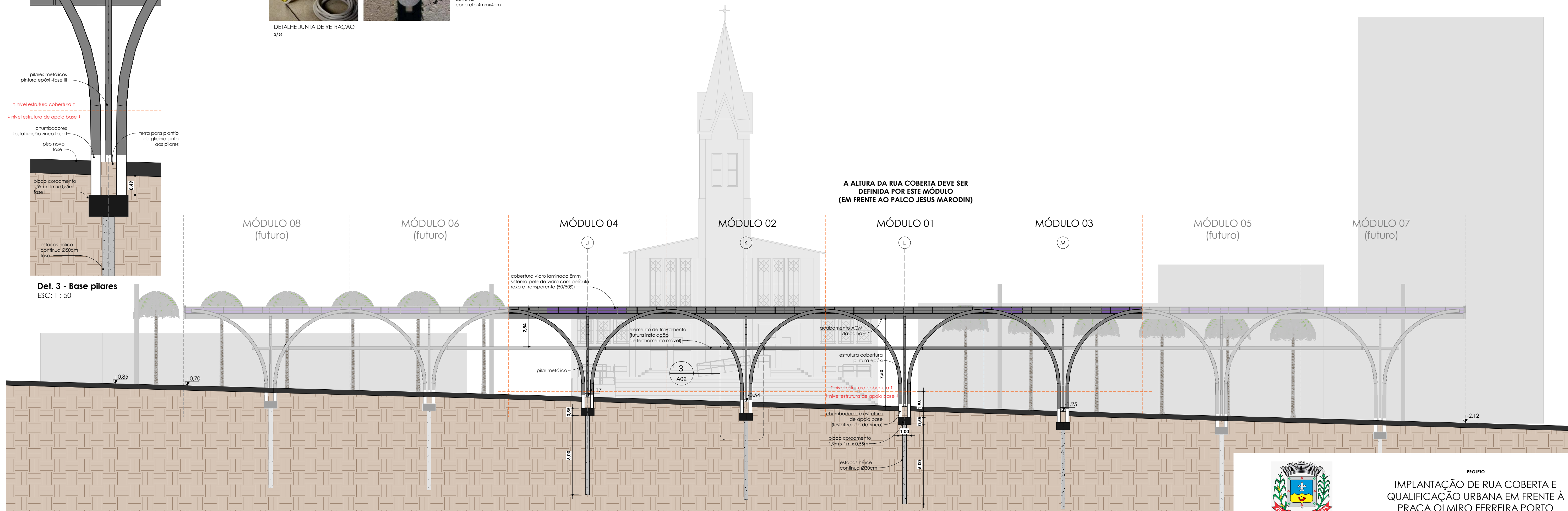
Corte "AA" ESC: 1 : 150
