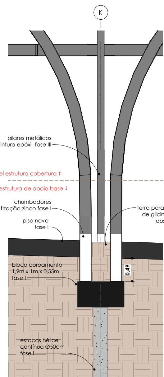
Det. 3 - Base pilares ESC: 1 : 50
