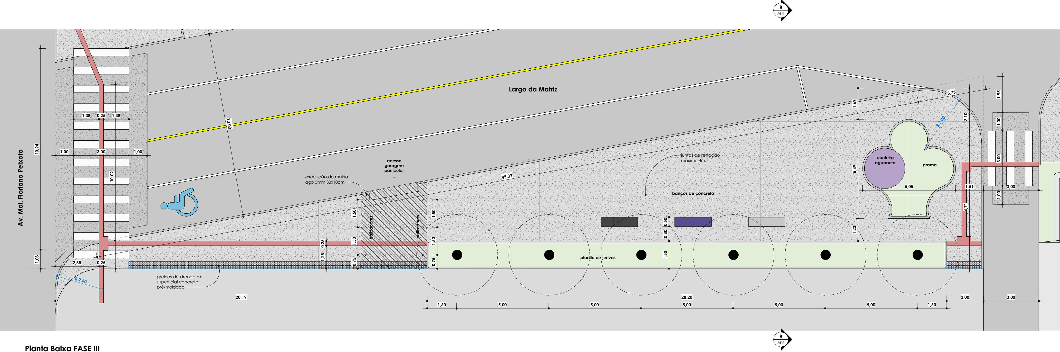
Planta Baixa FASE III ESC: 1 : 100
