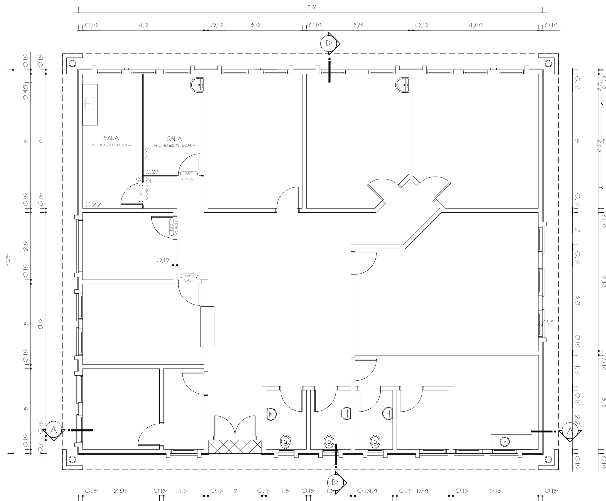
PLANTA BAIXA Escala 1/50
