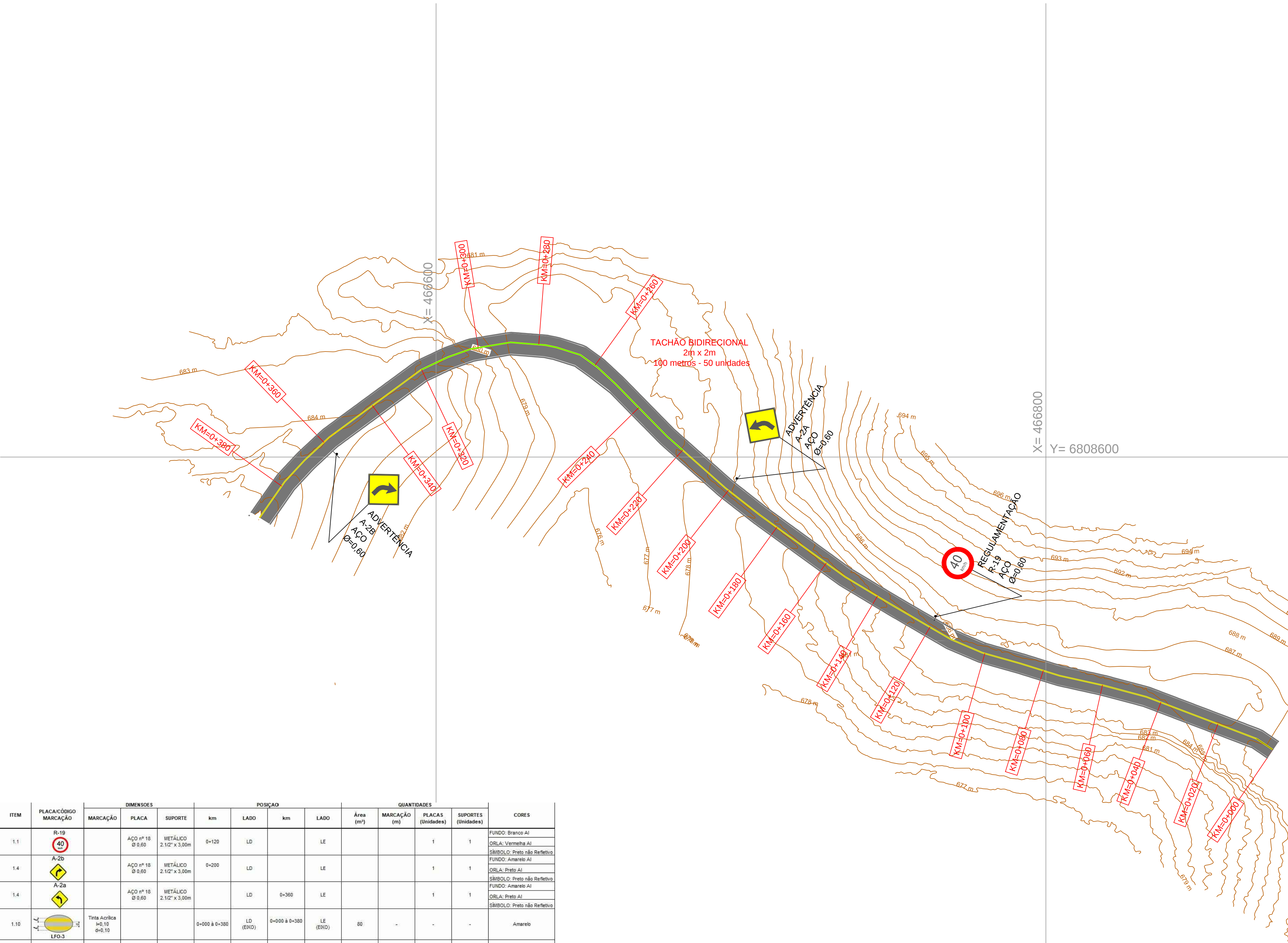
PROJETO DE SINALIZAÇÃO ESC.: 1:750
