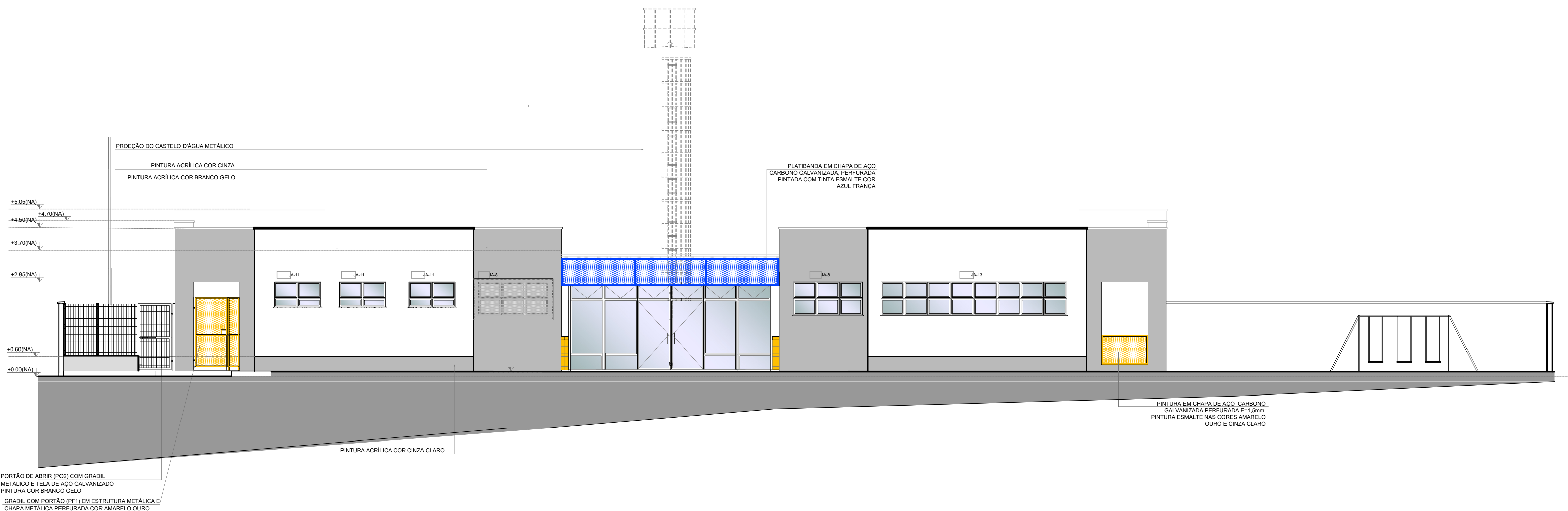
2 FACHADA NORTE ESCALA 1/75
