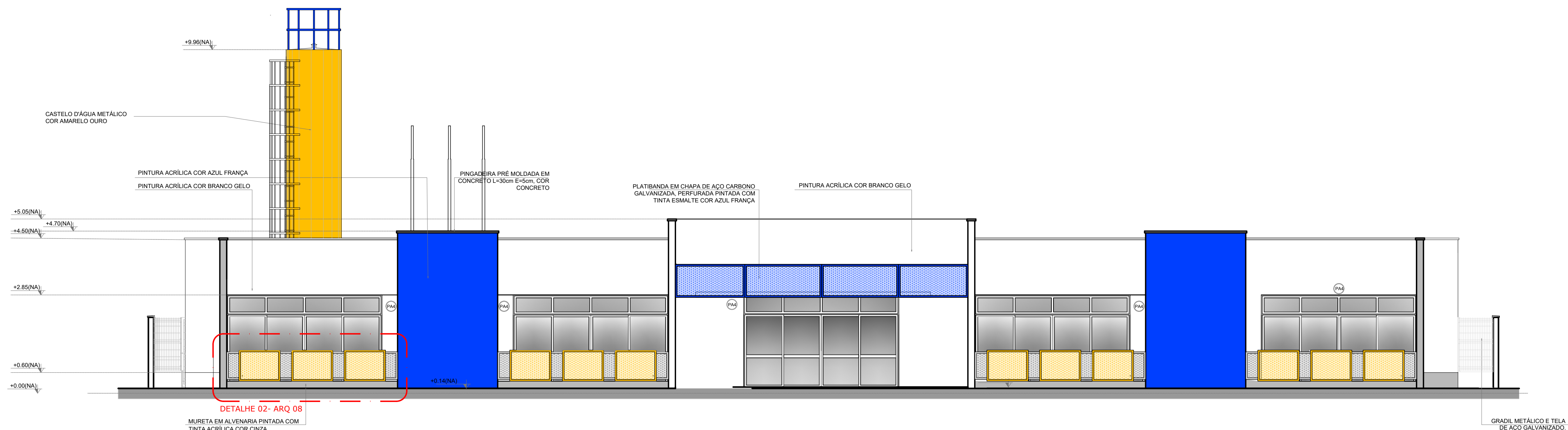
3 FACHADA OESTE ESCALA 1/75
