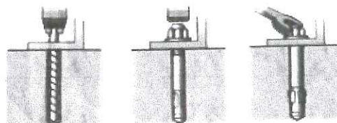
Furação, posicionamento e fixação.
