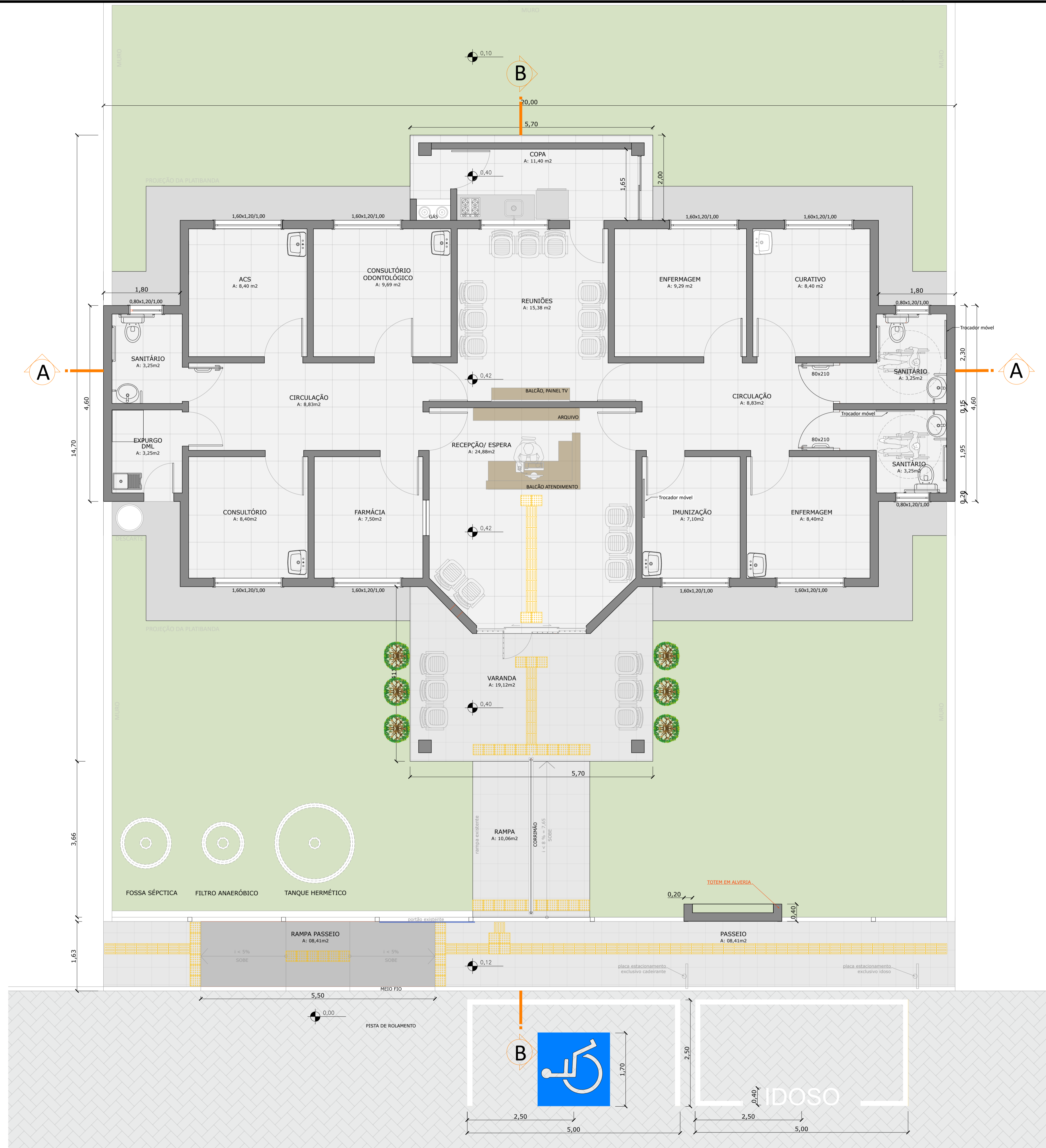
PLANTA BAIXA - LAYOUT ESC.:1/50
