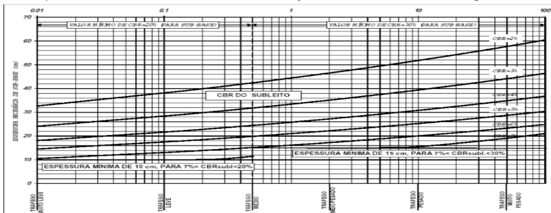
Figura 3 – Espessura mínima necessária de sub-base em função do CBR do subleito e do tráfego.
