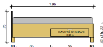
VISTA LATERAL
