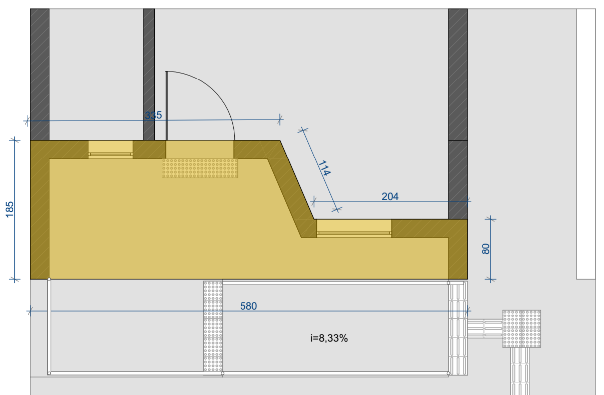
RECUERAÇÃO DE LAJE SUPERIOR ESC 1/50
