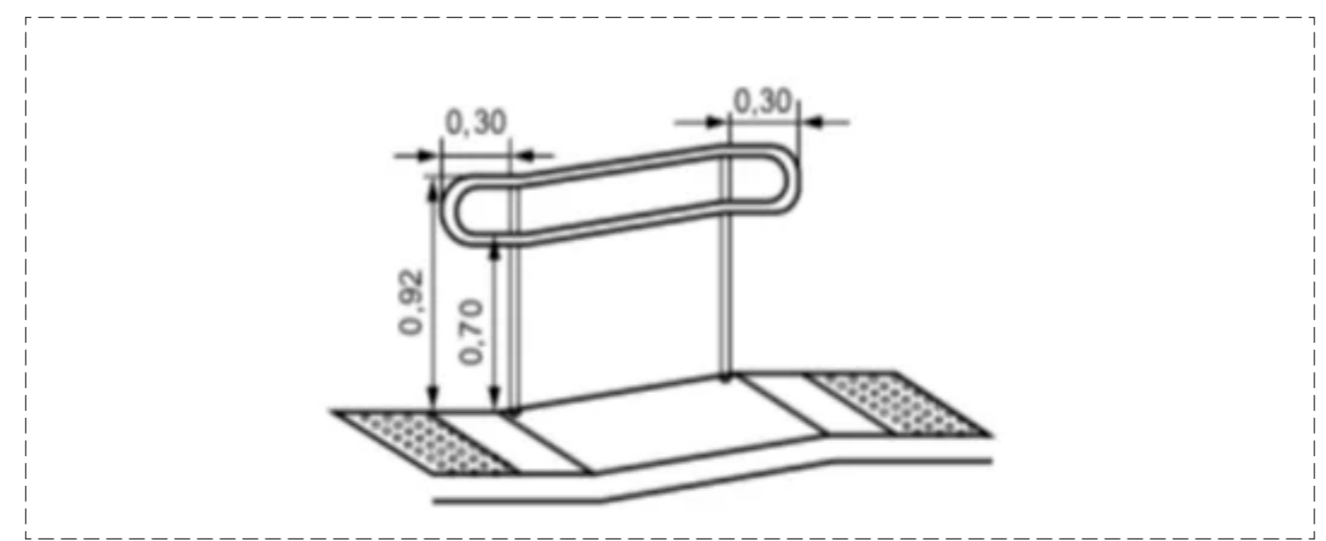
DETALHE CORRIMÃO
