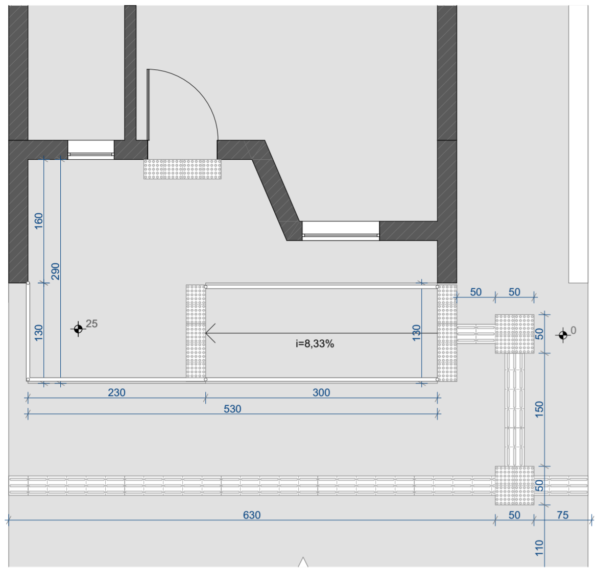
TÉRREO/RAMPA ESC 1/50
