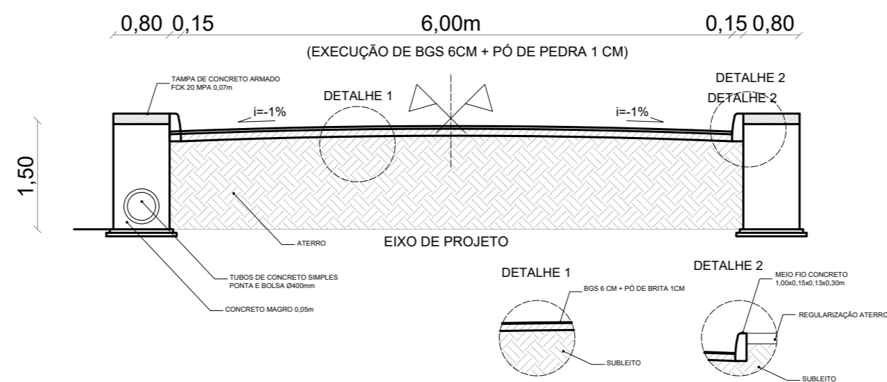
SEÇÃO TIPO ESCALA: 1/75
