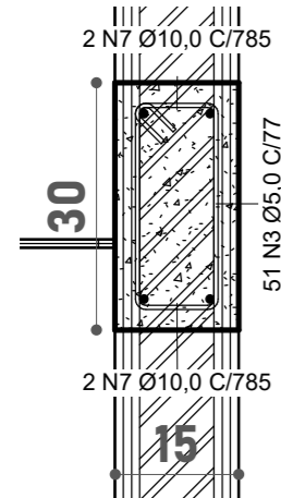
7 VIGAS V01-V06 1:10
