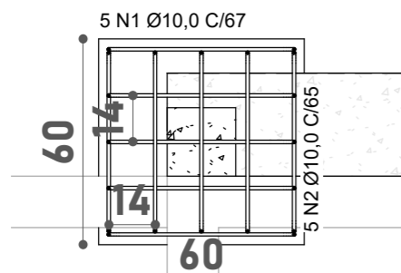
4 Sapata S1-S13 1:20
