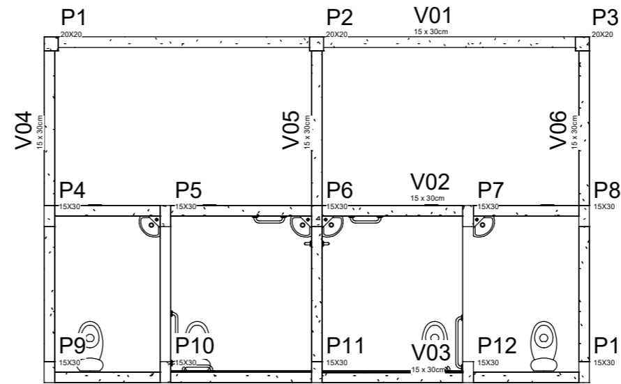
2 PÁV. SUPERIOR 1:75
