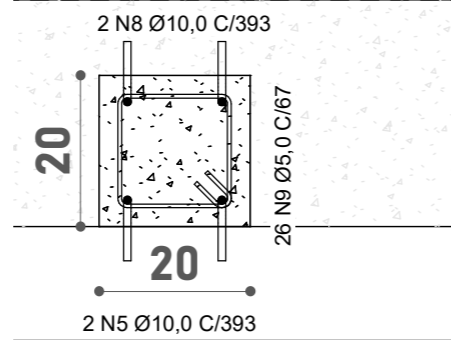
5 PILAR P1-P3 1:10
