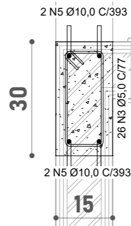
6 PILAR P4-P13 1:10
