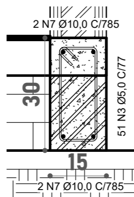
8 VIGAS VB01-V05 1:10
