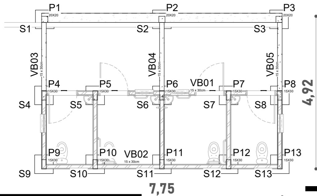
1 CALÇADA 1:75
