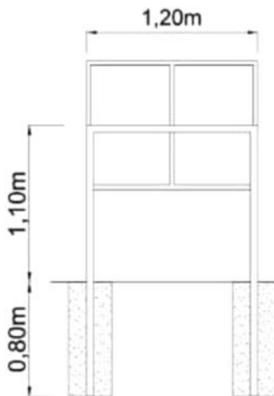
DETALHAMENTO PORTERIOR (quadro de perfil retangular 50mm x 30mm #2mm, fixado com braçadeiras ao suporte de tubo de aço 2")
