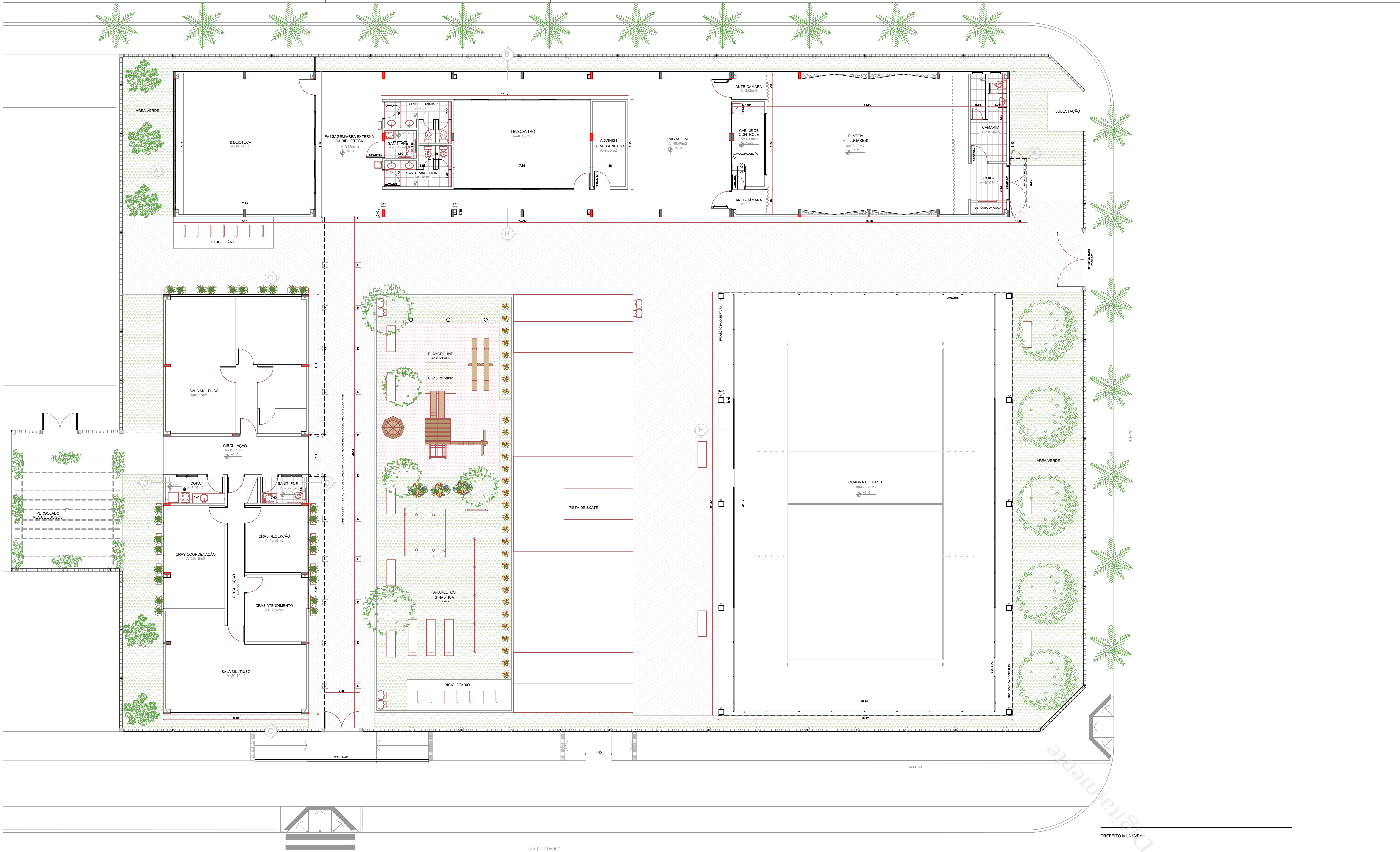
PLANTA BAIXA TÉRREO esc.: 1:100
