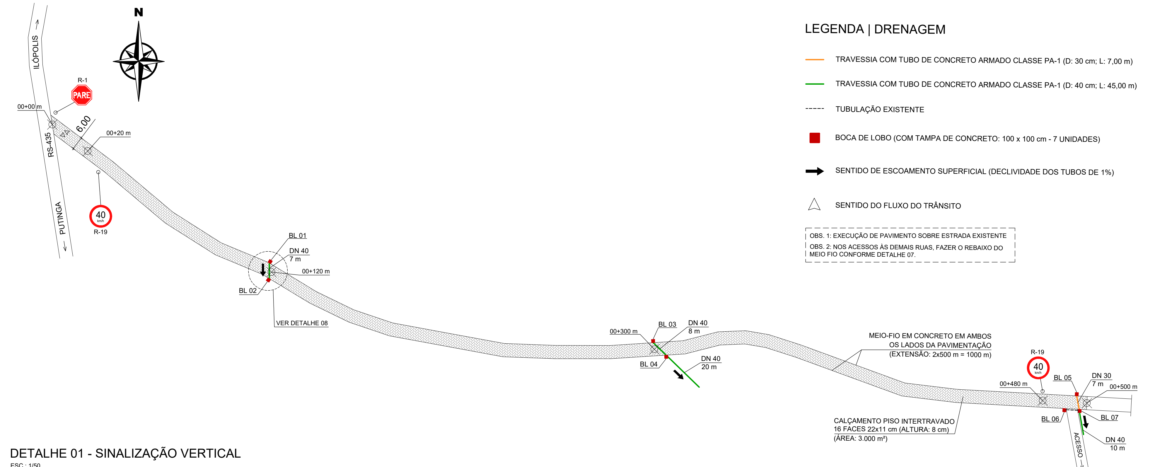
DRENAGEM E SINALIZAÇÃO_PAV. MARIA QUITÉRIA EXTENSÃO: 500 m ESC.: 1/1000
