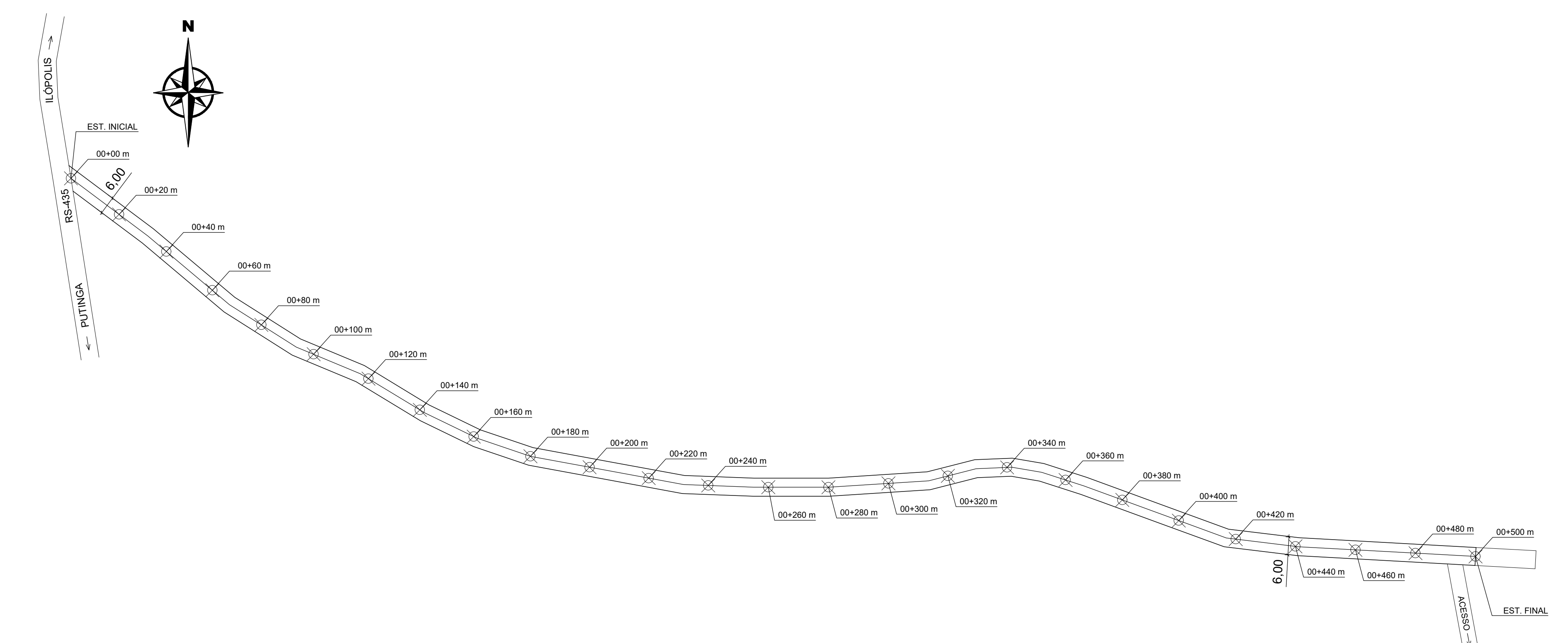
PLANIMETRIA_PAV. MARIA QUITÉRIA EXTENSÃO: 500 m ESC.: 1/1000
