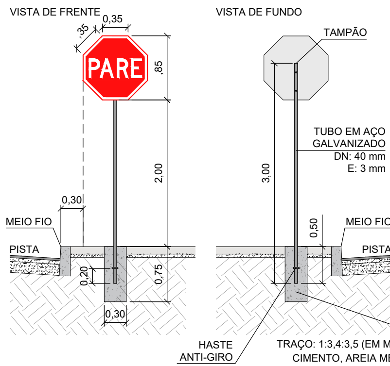
DETALHE 01 - SINALIZAÇÃO VERTICAL ESC.: 1/50 (EM m)
