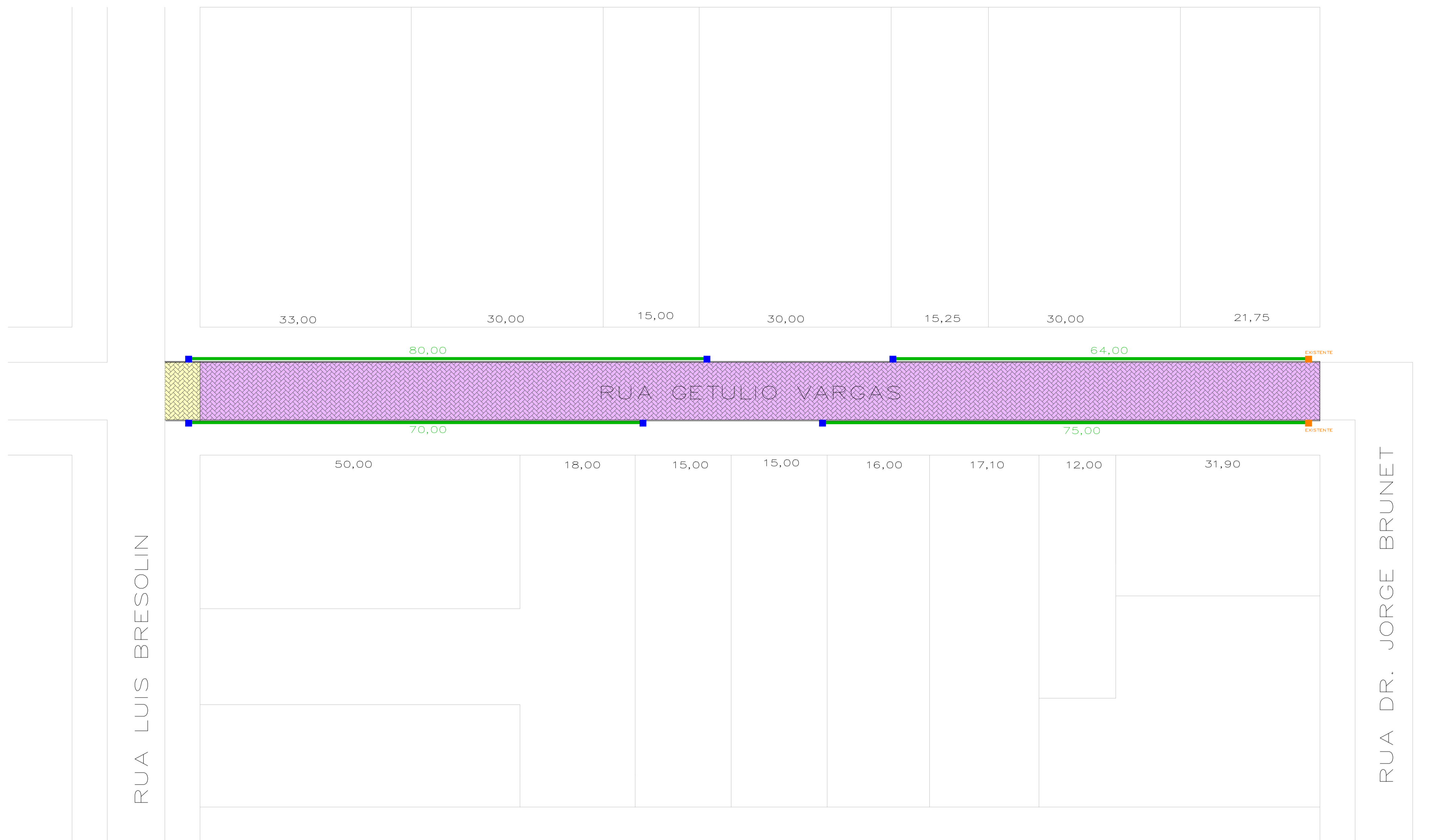
PLANTA BAIXA PAV. E DRENAGEM RUA GETÚLIO VARGAS - TRECHO 2 ESC.: 1/400
