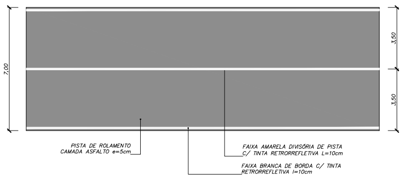
DETALHE SINALIZAÇÃO 1/75
