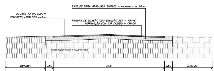
SEÇÃO TRANSVERSAL 1/20
