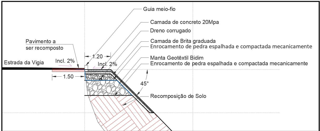
Detalhe Recomposição de encosta – enrocamento de pedra
