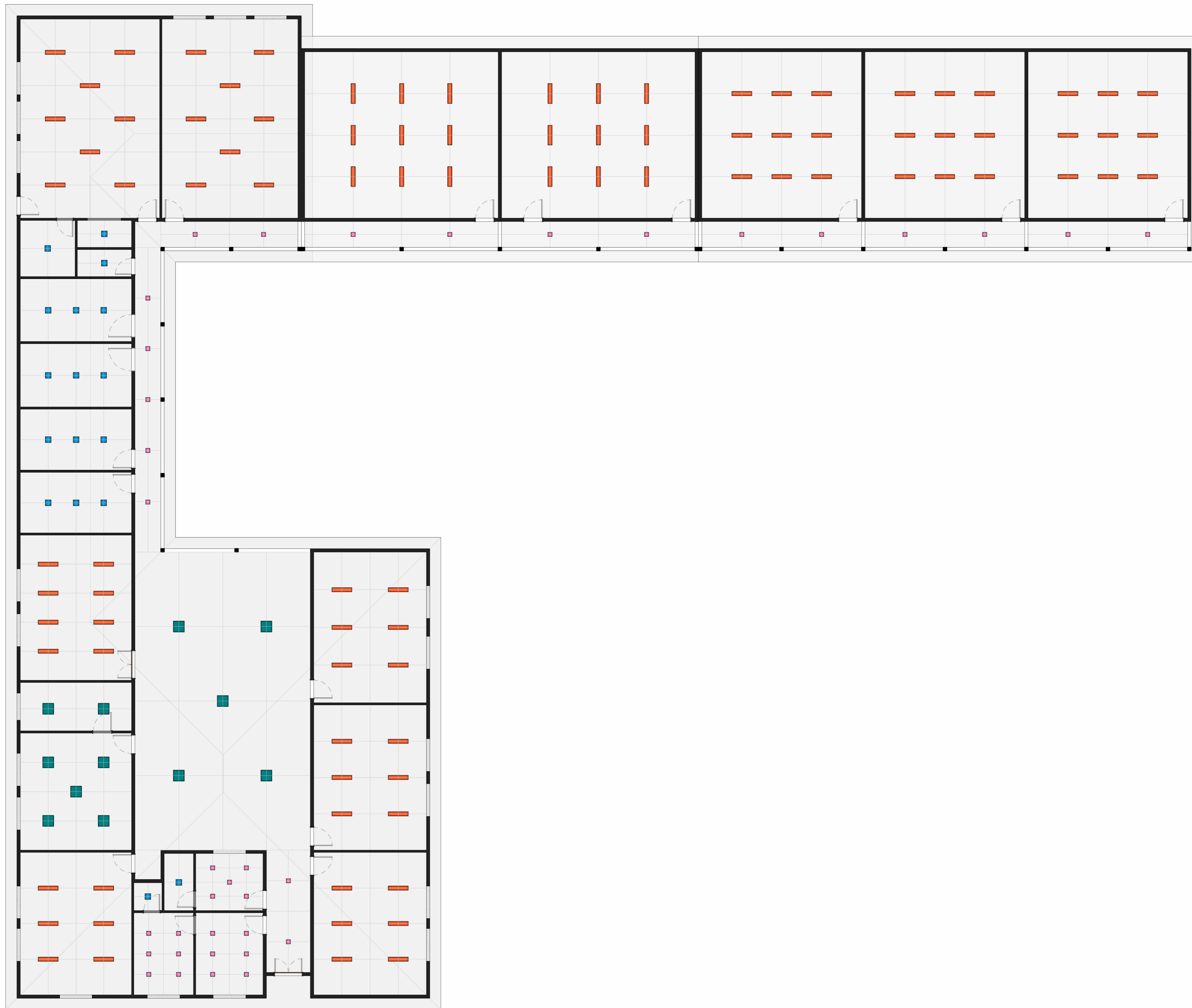
01 PLANTA DE FORRO - LUMINOTÉCNICO Escala: 1:100
