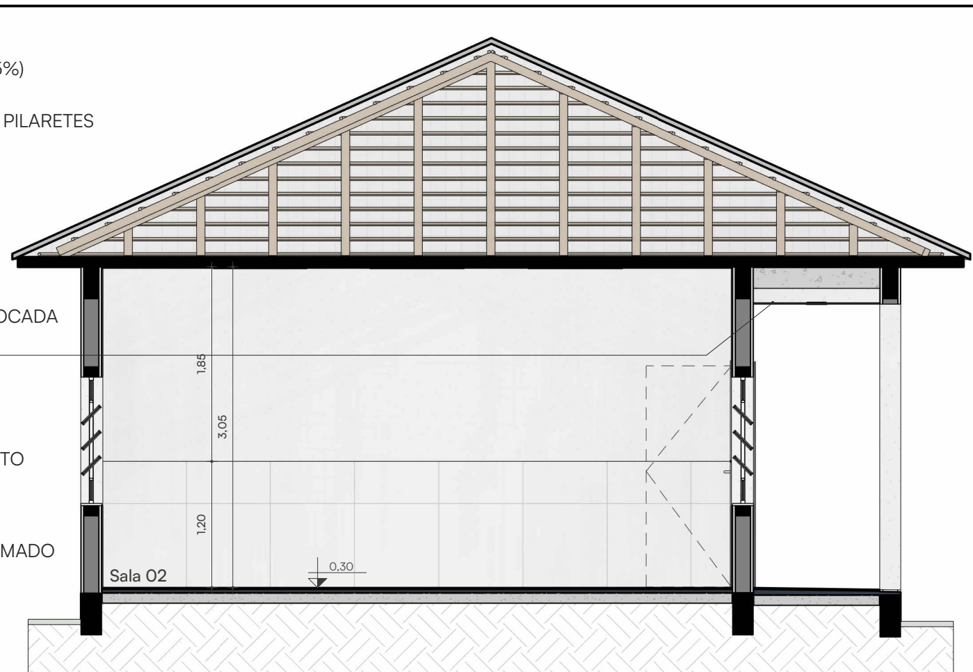
02 CORTE - B' Escala: 1:50
