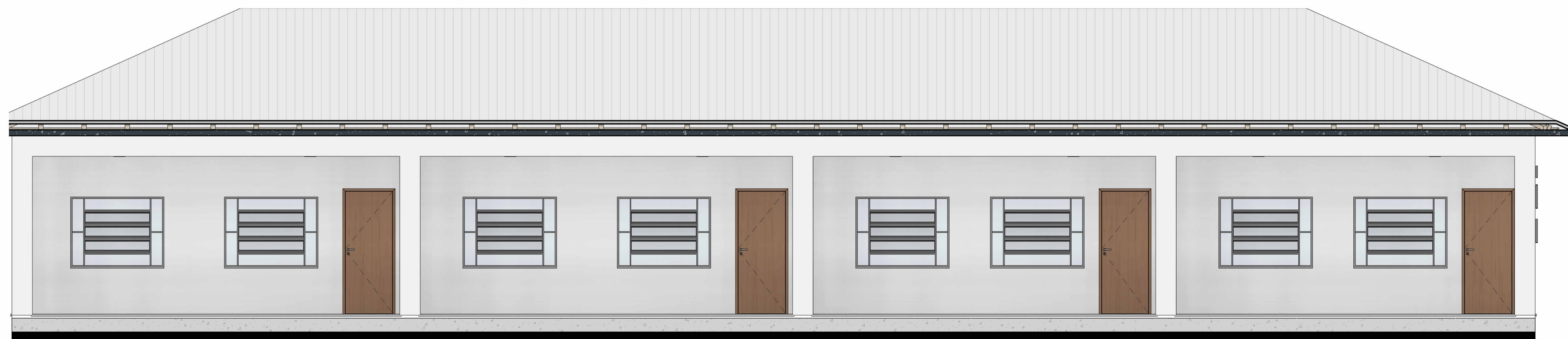
03 FACHADA - LATERAL ESQUERDA Escala: 1:50
