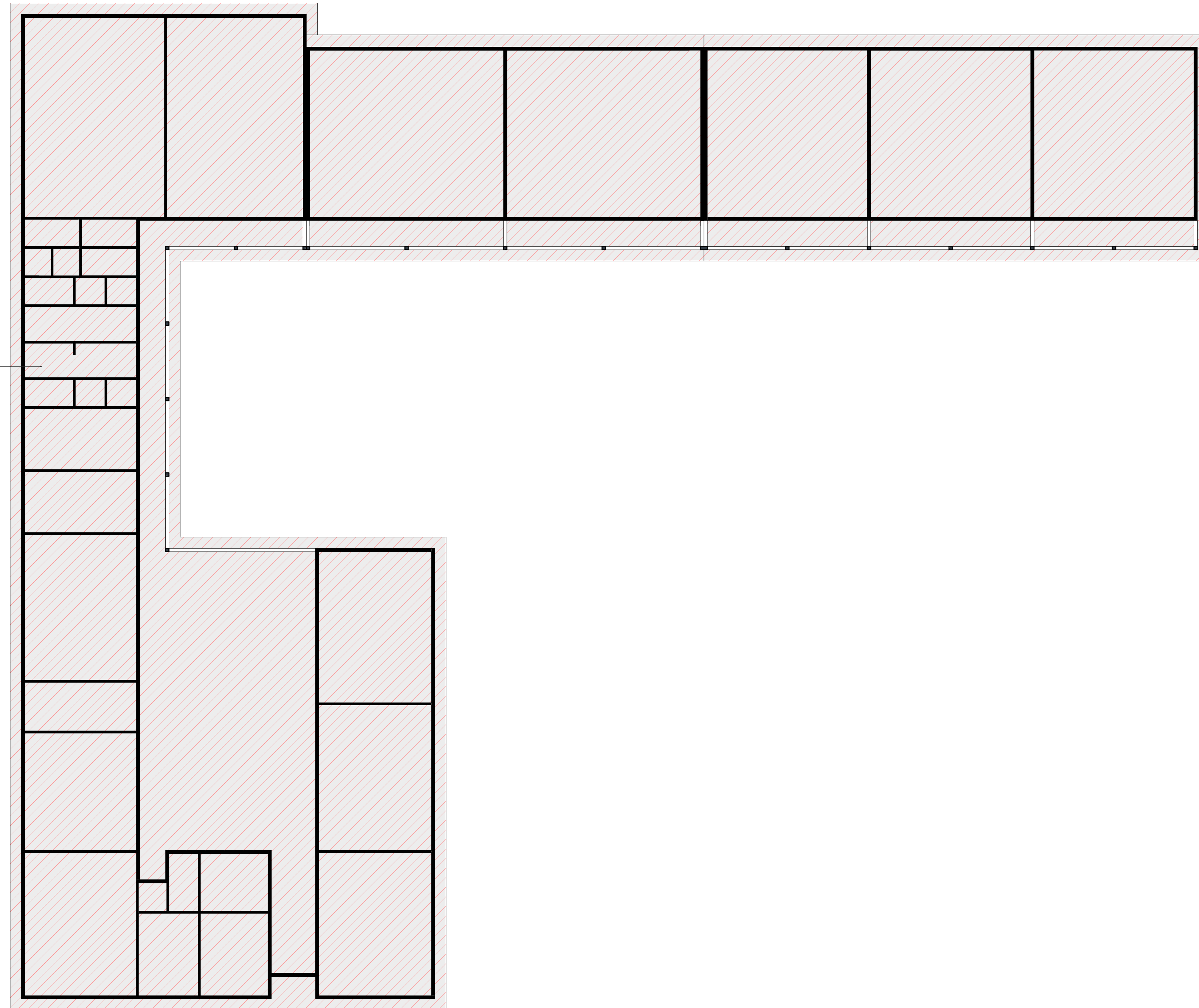
01 PLANTA DE FORRO - CONSTRUIR Escala: 1:100
