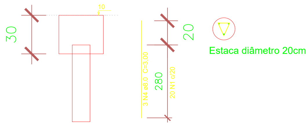
DETALHAMENTO BLOCO E ESTACA
