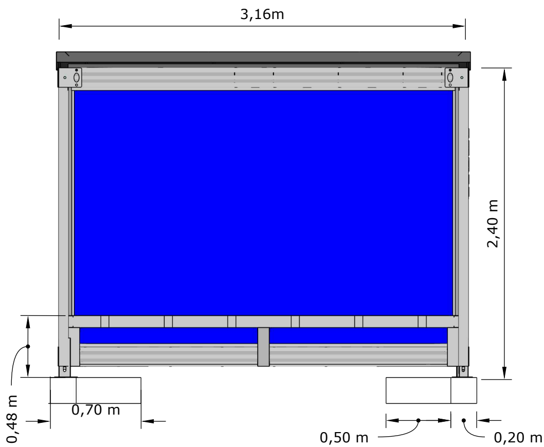
Vista frontal escala 1:30
