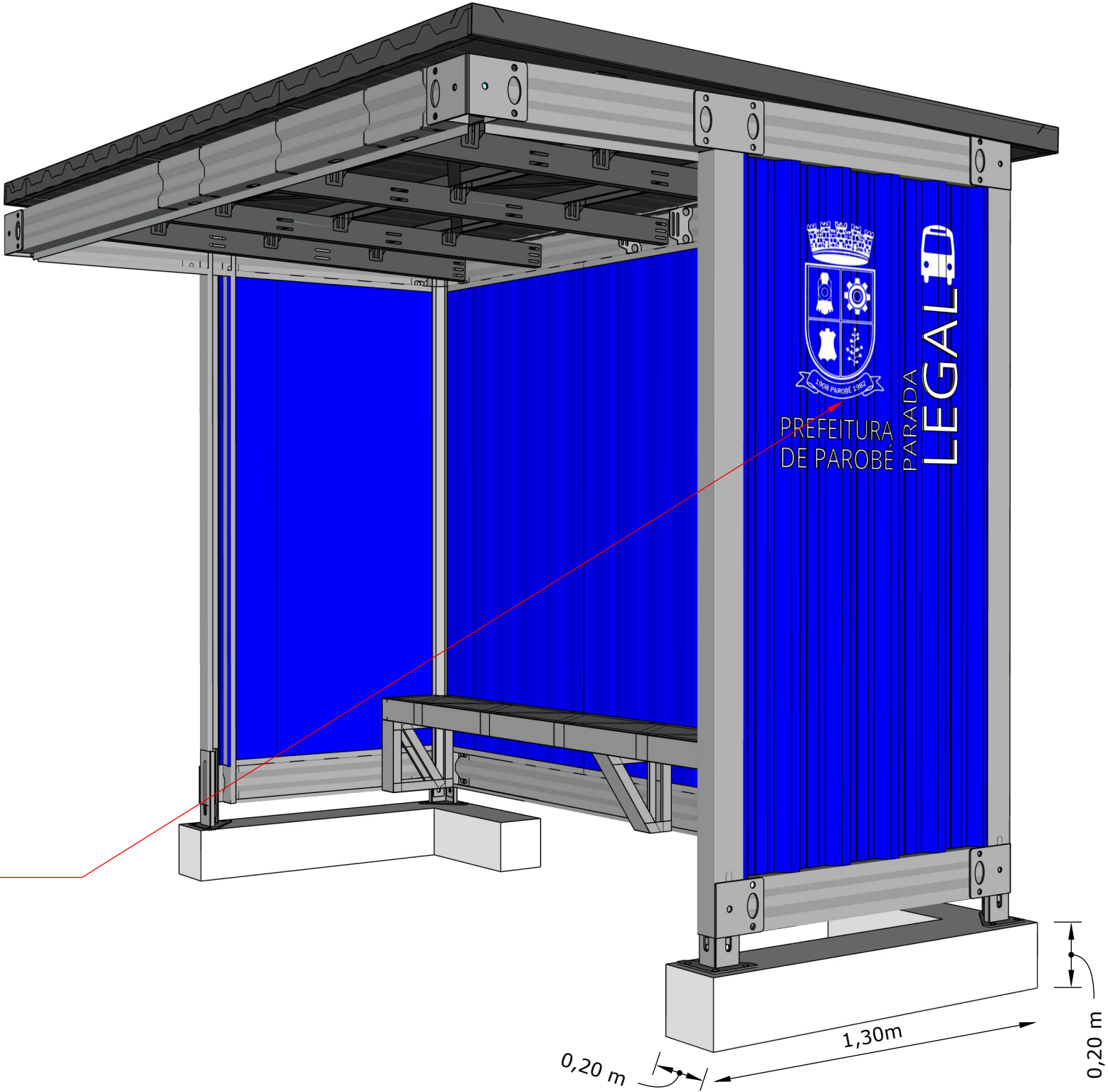
Esquema isométrico sem escala
