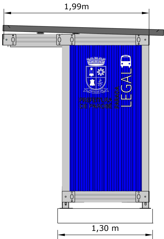
Vista Lateral Direita escala 1:30
