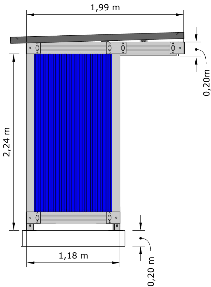
Vista Lateral Esquerda escala 1:30
