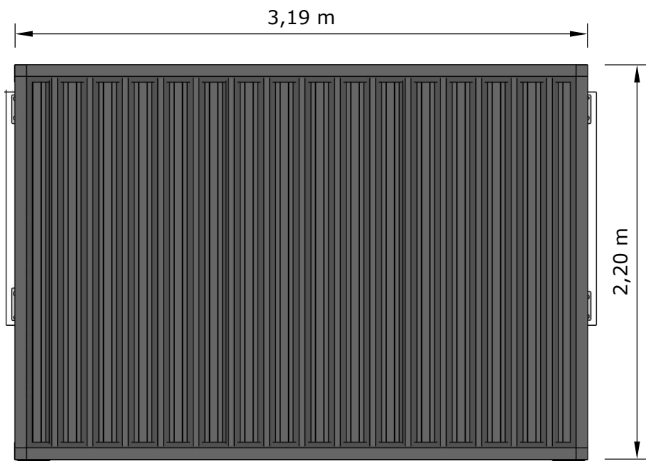
Vista superior escala 1:30
