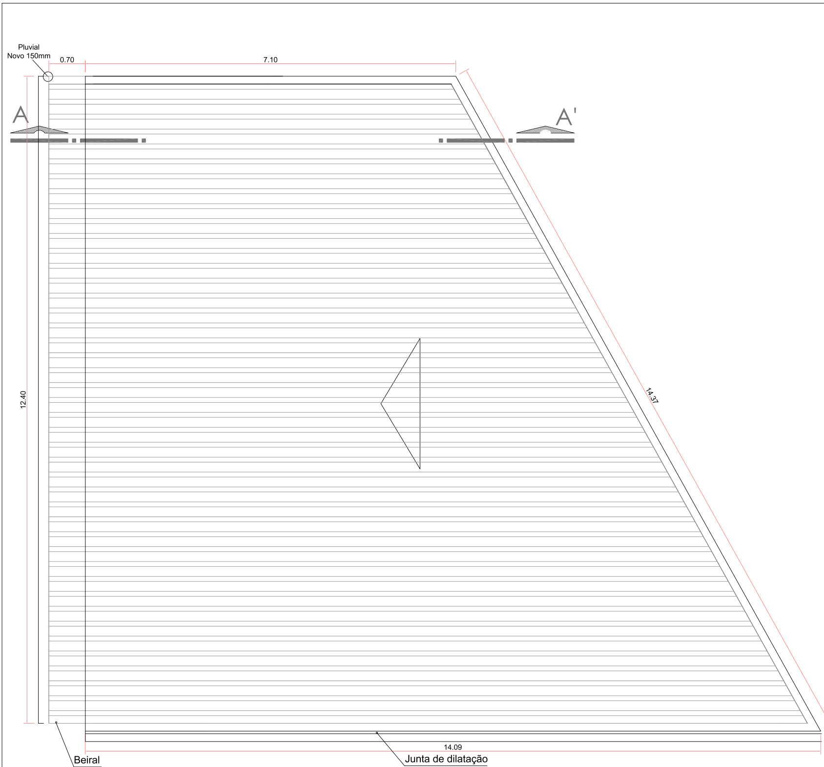
Planta de Cobertura Esc.1/50 Área: 135,00
