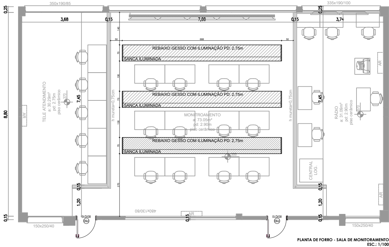
PLANTA DE FORRO - SALA DE MONITORAMENTO ESC.: 1/100
