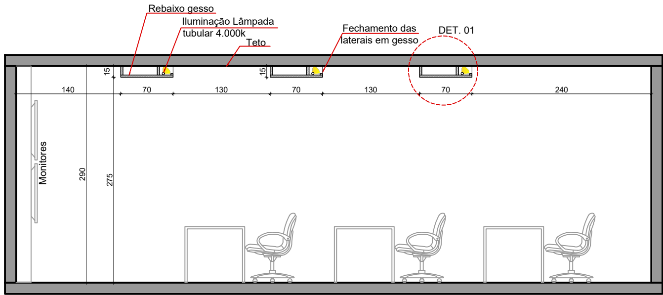
VISTA LATERAL - SALA DE MONITORAMENTO ESC.: 1/50
