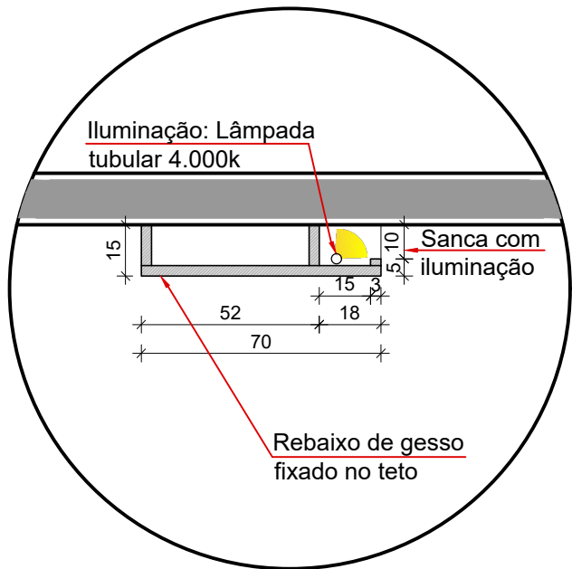
DETALHE 01- REBAIXO DE GESSO COM ILUMINAÇÃO ESC.: 1/20
