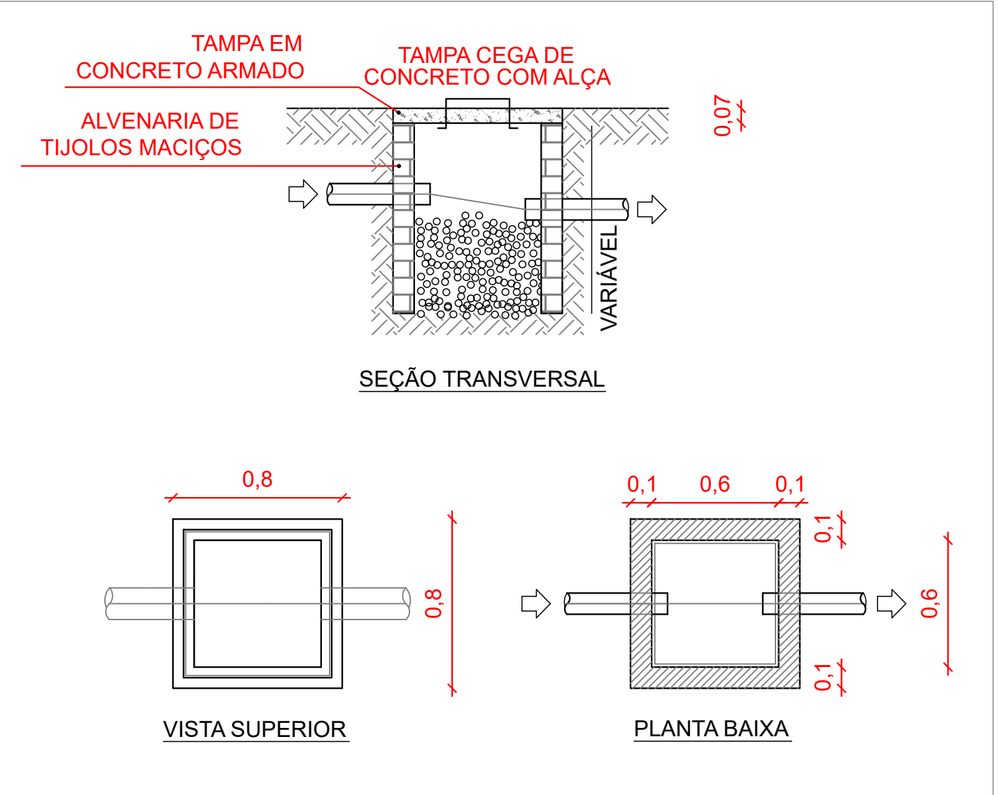
02 DETALHAMENTO - CAIXAS Escala: 1/25
