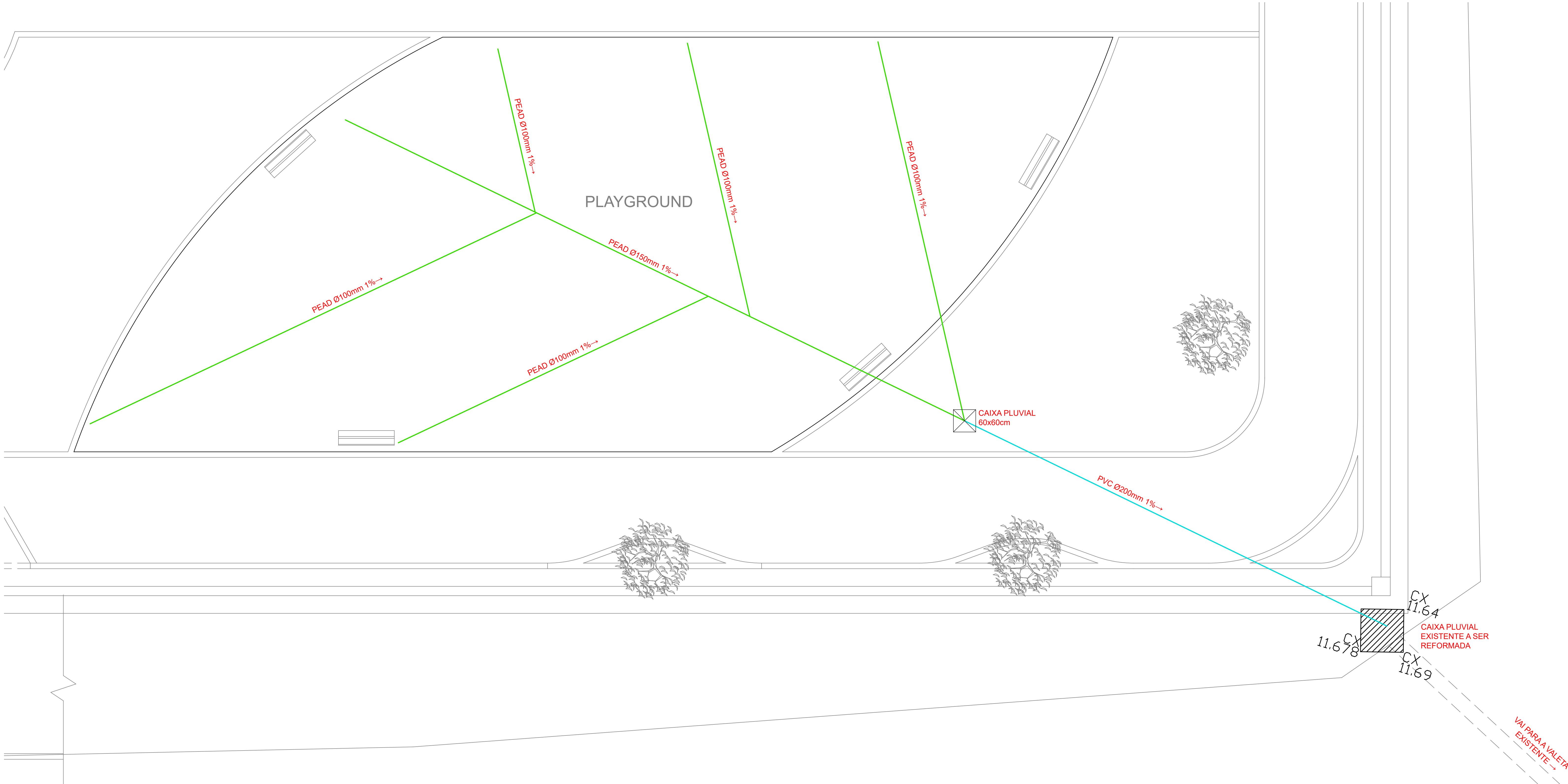
01 DRENAGEM DO PLAYGROUND Escala: 1/100
