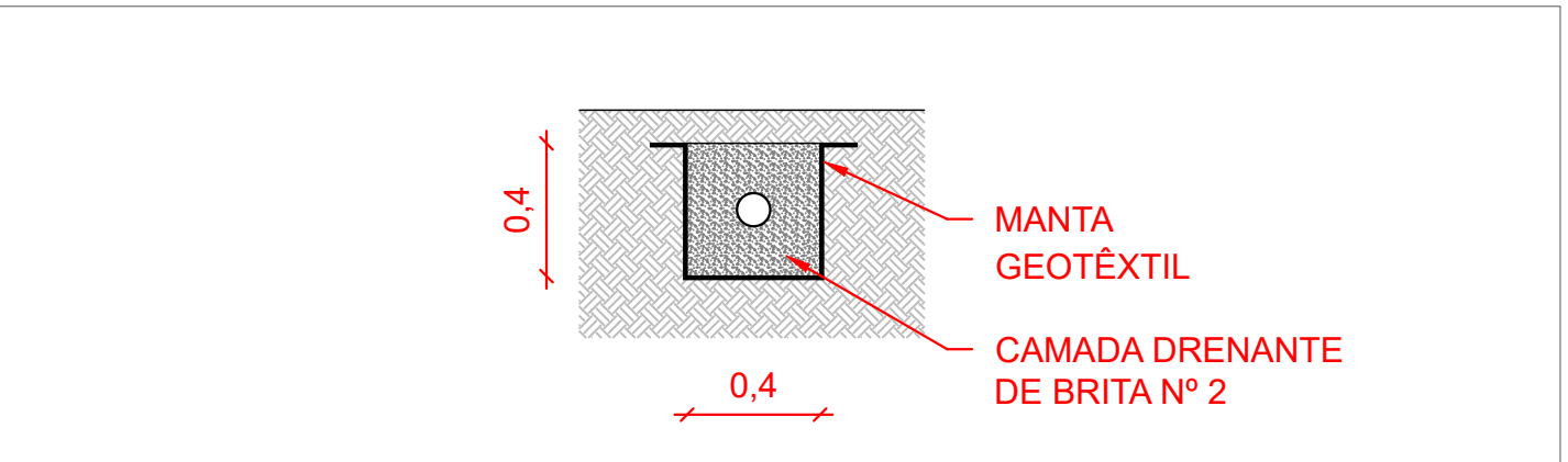
03 DETALHAMENTO - MANTA GEOTÊXTIL Escala: 1/25
