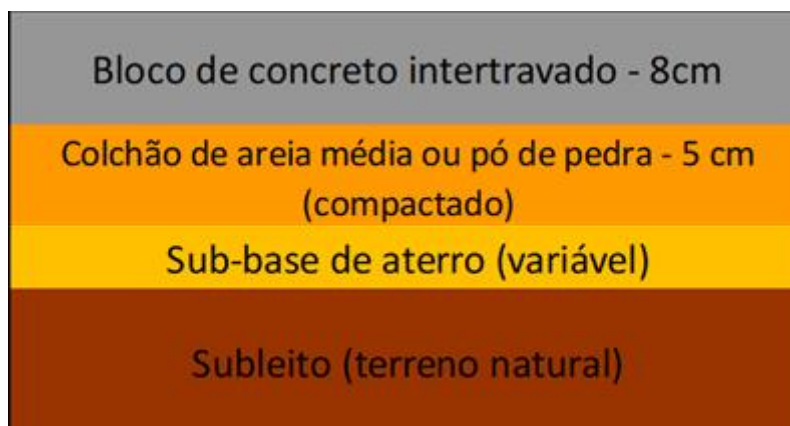
Figura 12 - Camadas pavimento com blocos de concreto intertravado
