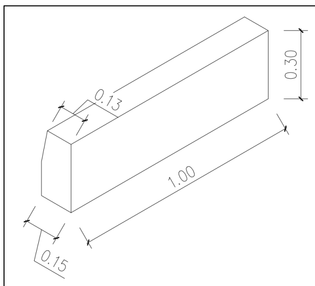
Figura 11 - Desenho esquemático do meio-fio
