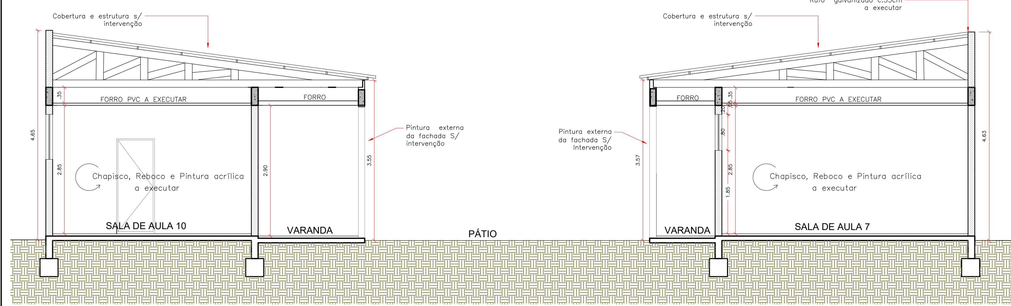
04 CORTE CC' - A CONSTRUIR ESCALA 1:50
