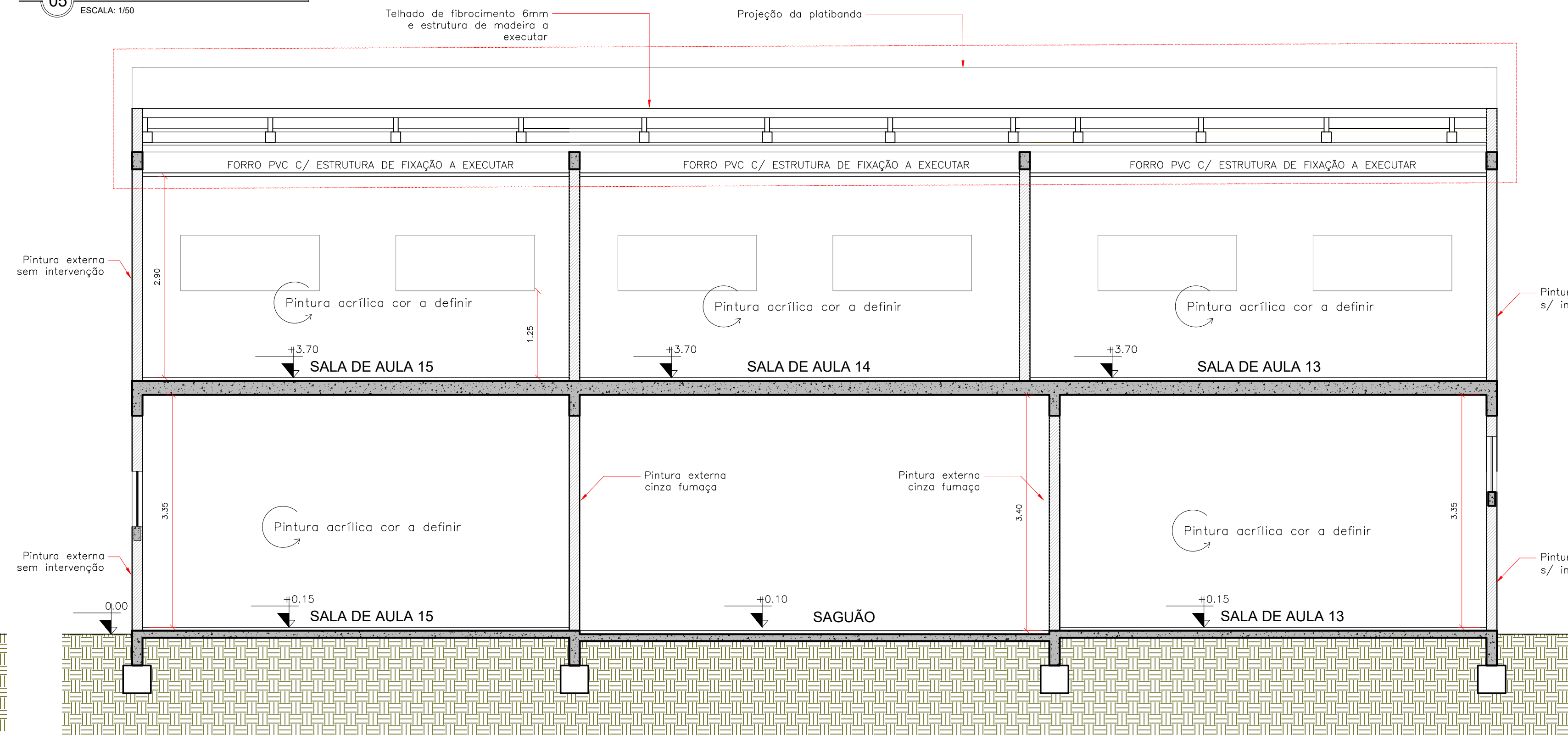
06 CORTE AA' - A CONSTRUIR ESCALA 1:50
