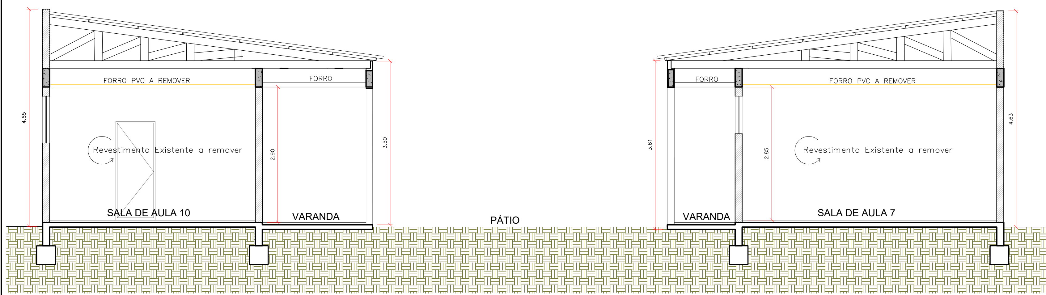
03 CORTE CC' - A REMOVER ESCALA 1:50
