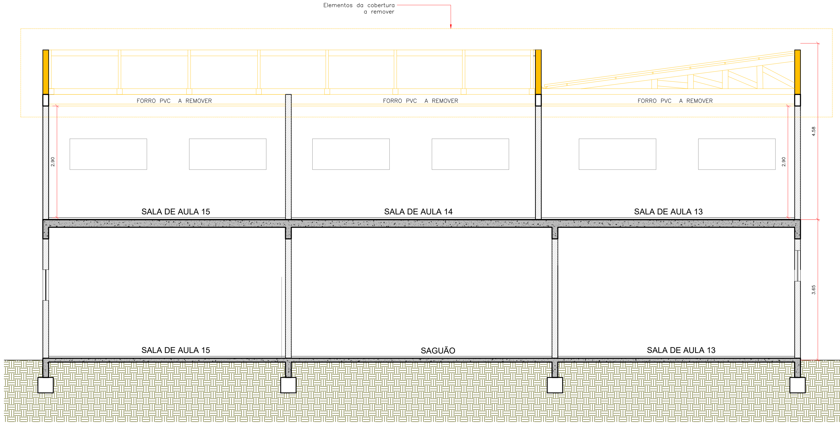
05 CORTE AA' - A REMOVER ESCALA 1:50
