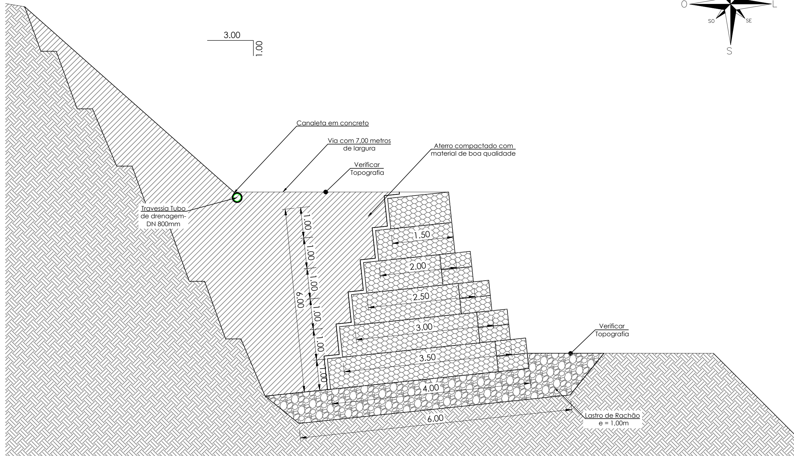
DETALHE DO MURO DE GABIÃO ESCALA 1/75
