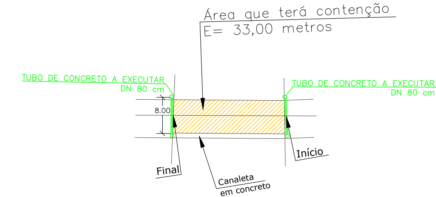
PLANTA BAIXA - TRECHO 03 SEM ESCALA
