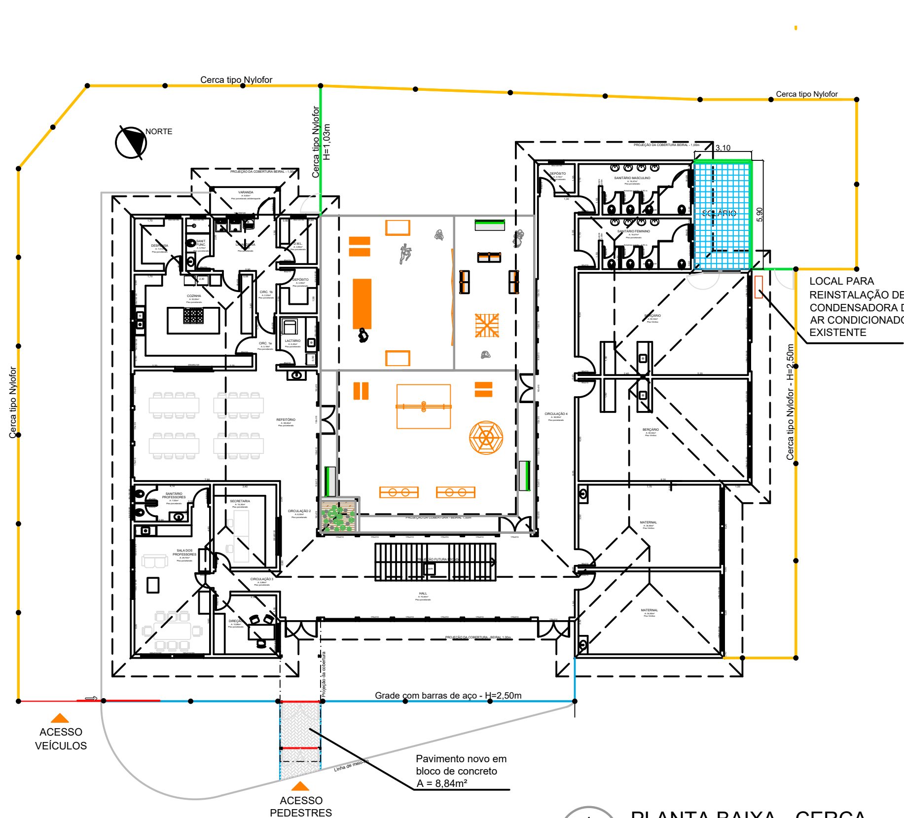
1 01 PLANTA BAIXA - CERCA Escala: 1/200
