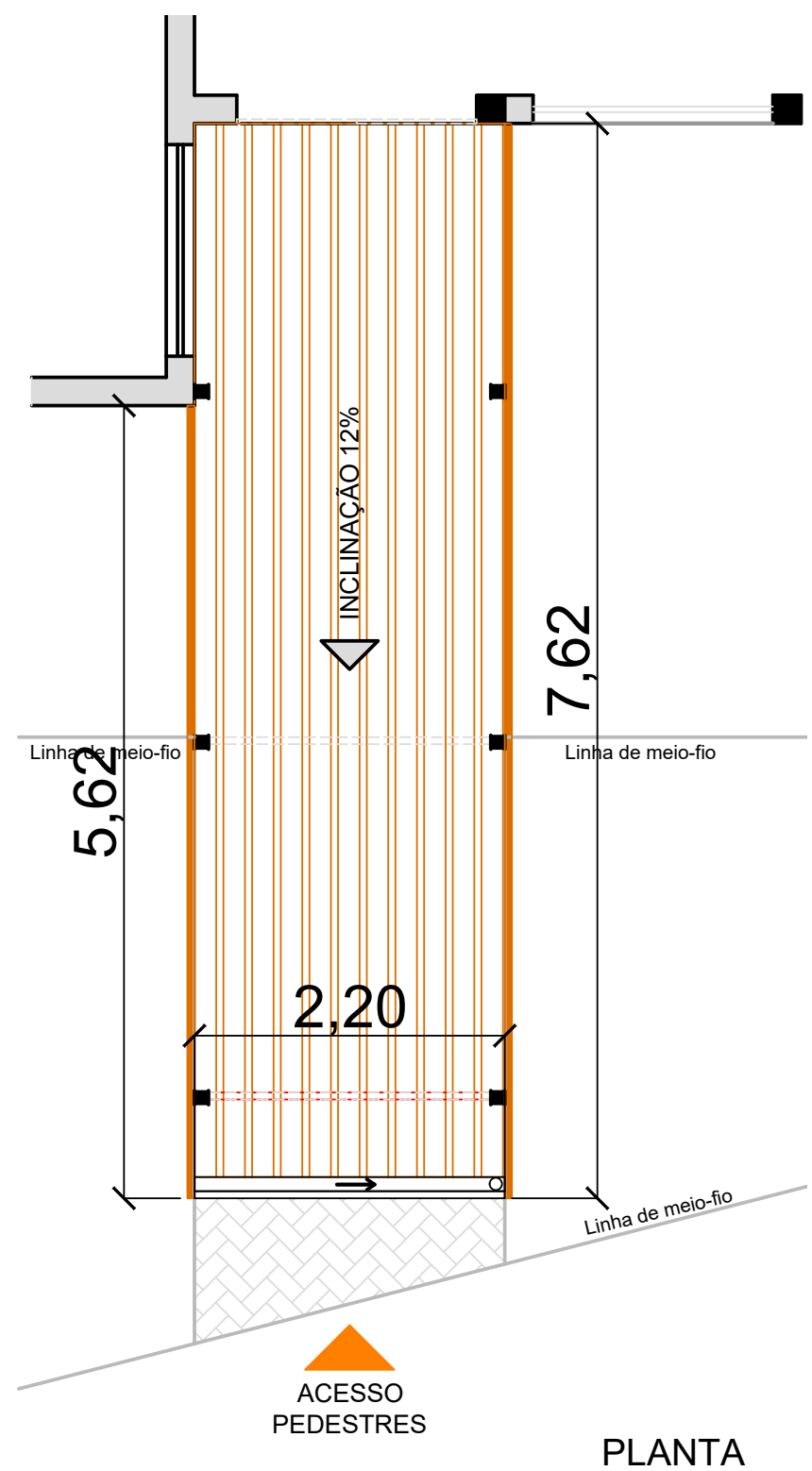
PLANTA
