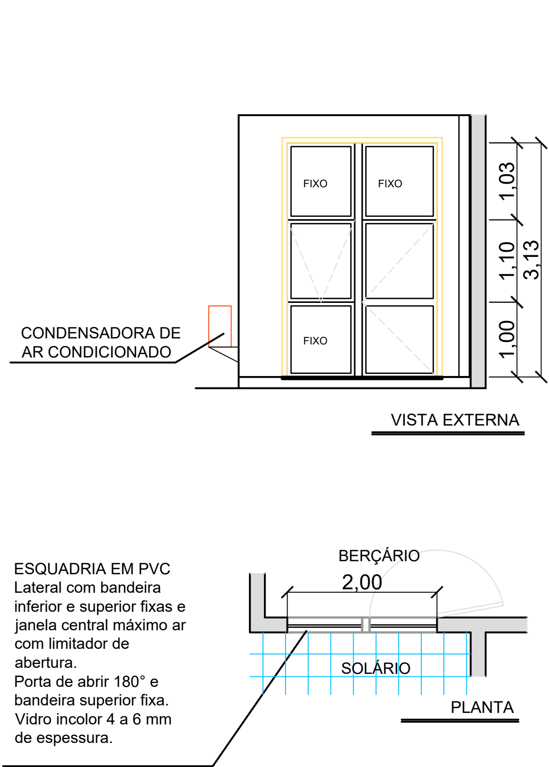
3 01 ESQUADRIA PVC Escala: 1/50
