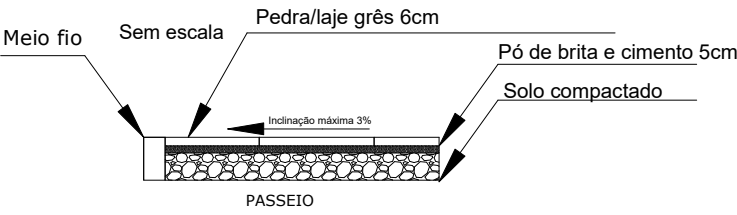
DETALHAMENTO DO MEIO FIO S/ ESCALA
