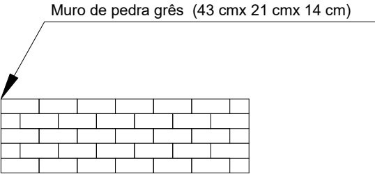
DETALHAMENTO MURO DE PEDRA GRÊS S/ ESCALA
