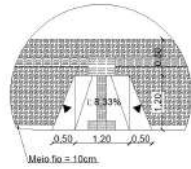
Figura 46 - Mudança de direção 150° < X ≤ 180°
