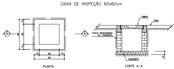
DETALHAMENTO CAIXA DE INSPEÇÃO S/ ESCALA
