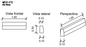
DETALHAMENTO DO MEIO FIO S/ ESCALA
