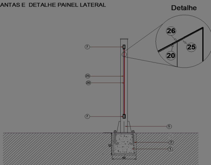
Detalhamento - Painel Lateral Módulo 1,82m x 3,00 m
