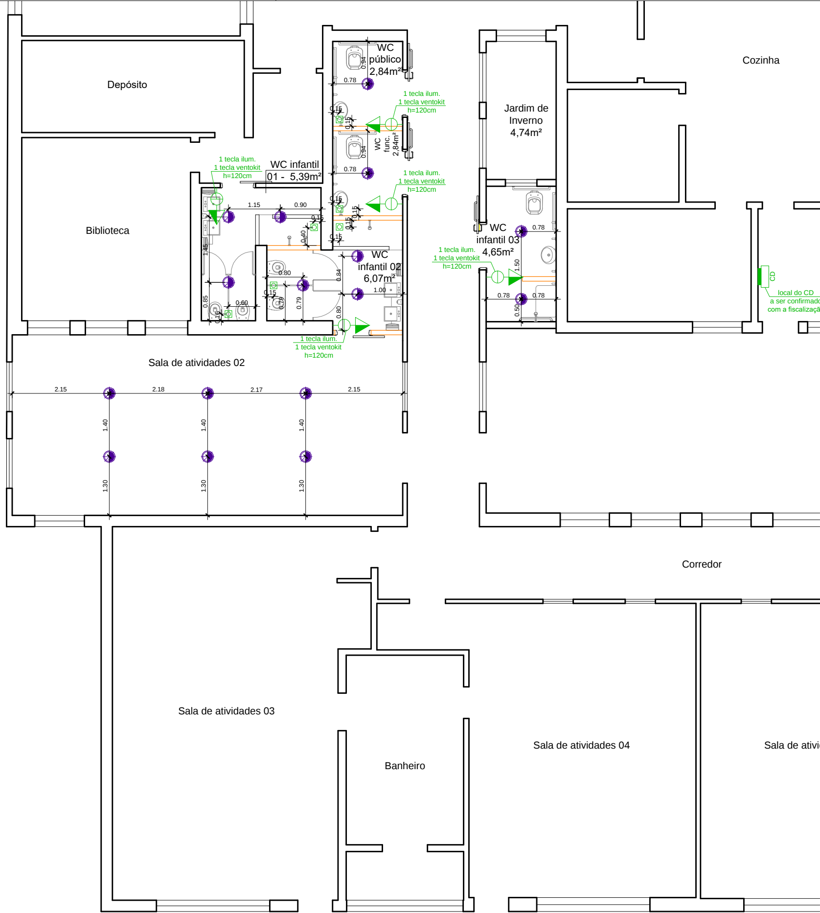
PLANTA BAIXA PONTOS ELÉTRICOS
