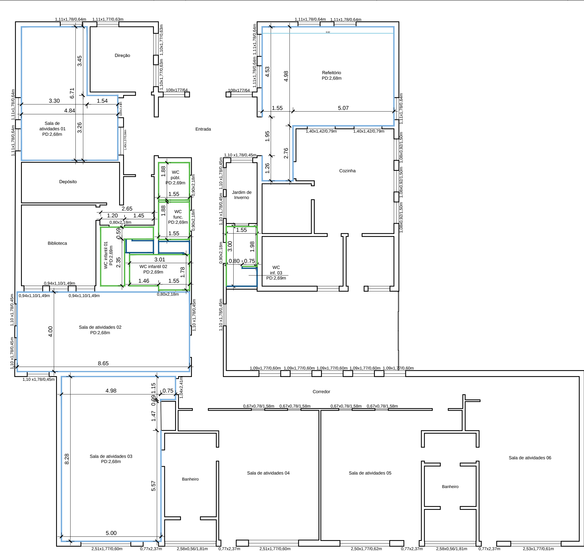
PLANTA BAIXA REVESTIMENTOS PAREDES INTERNAS
