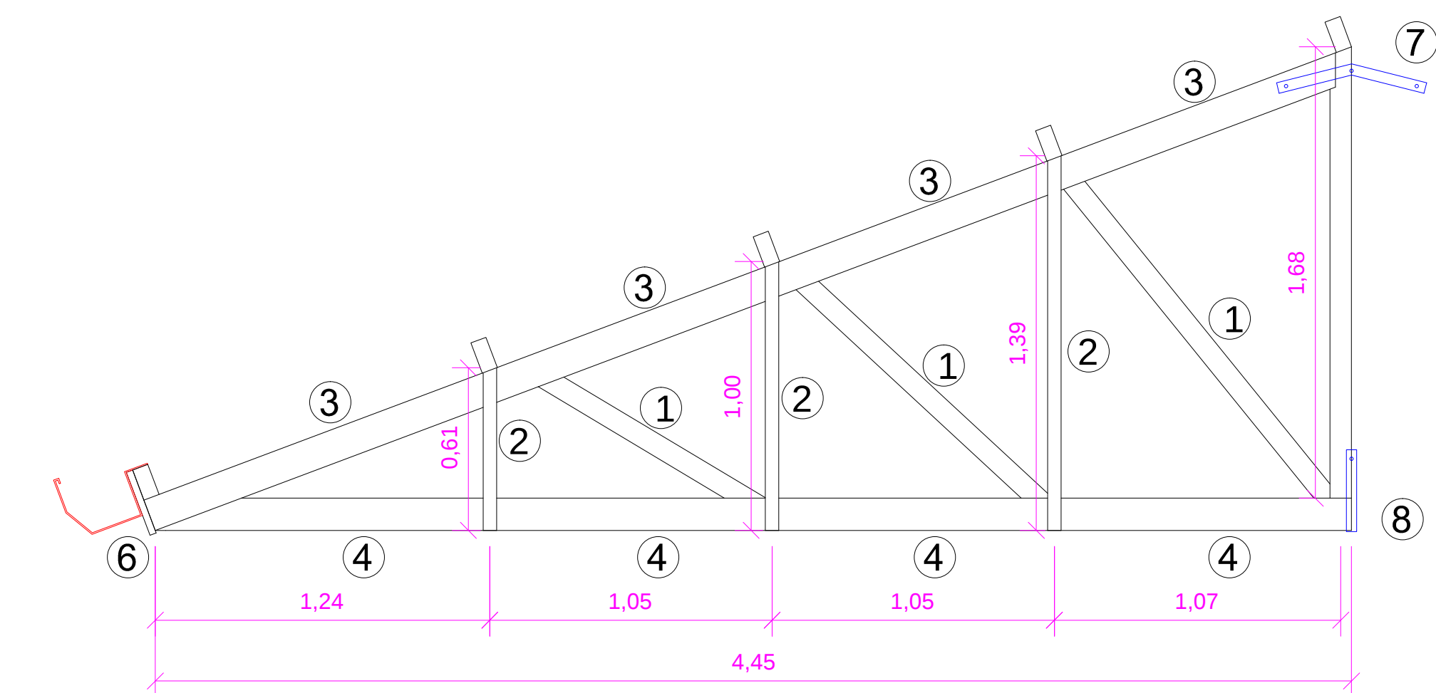
TESOURA 6, 7 ESC. 1/20
