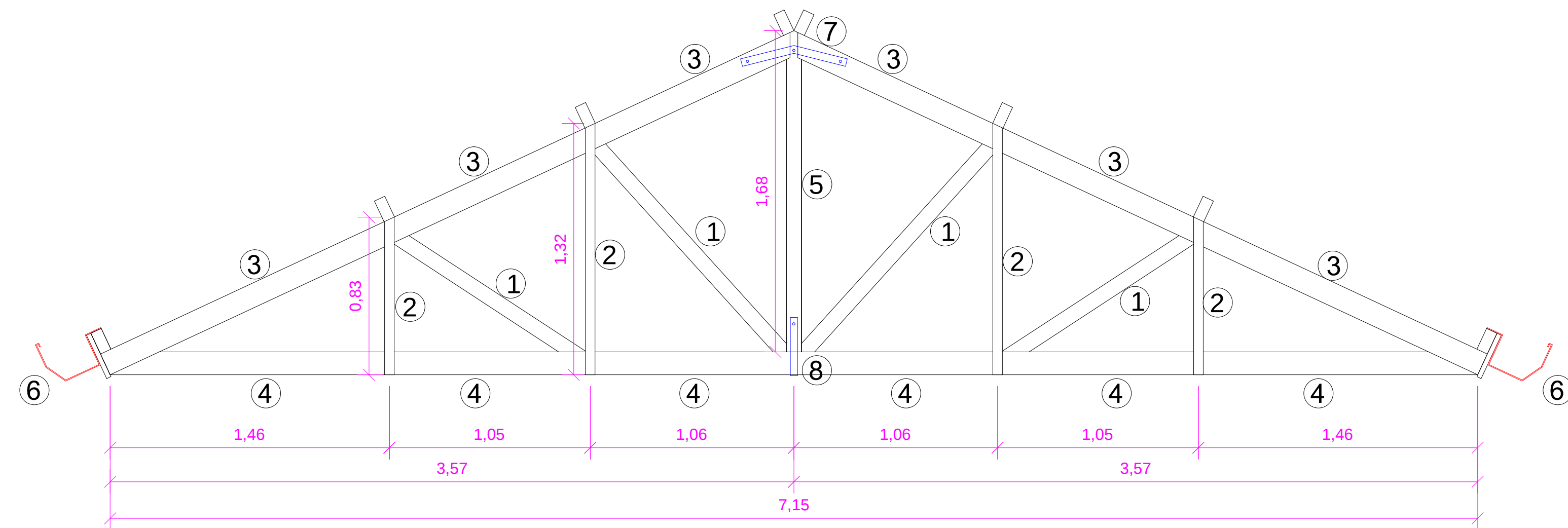
TESOURA 5 ESC. 1/20
