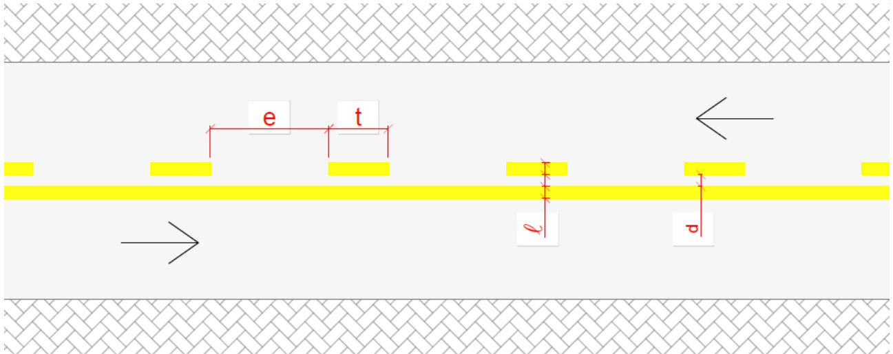
Figura 04 – Linha Dupla Contínua/Seccionada Amarela
