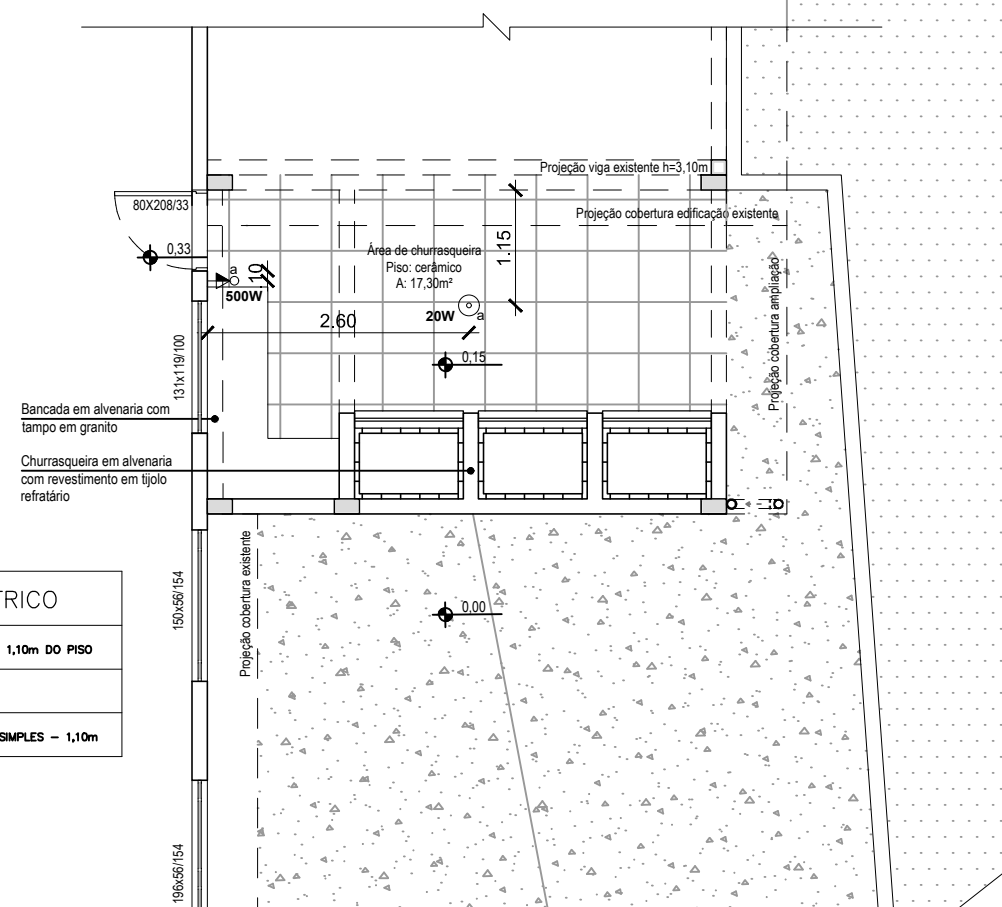
PLANTA ELÉTRICO Esc: 1/75
