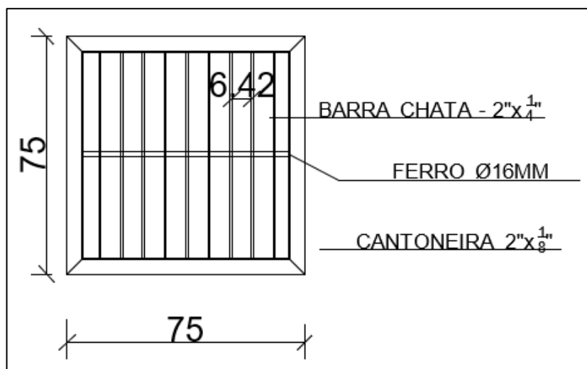
Figura 1 Detalhamento Grelha - Ferro redondo
