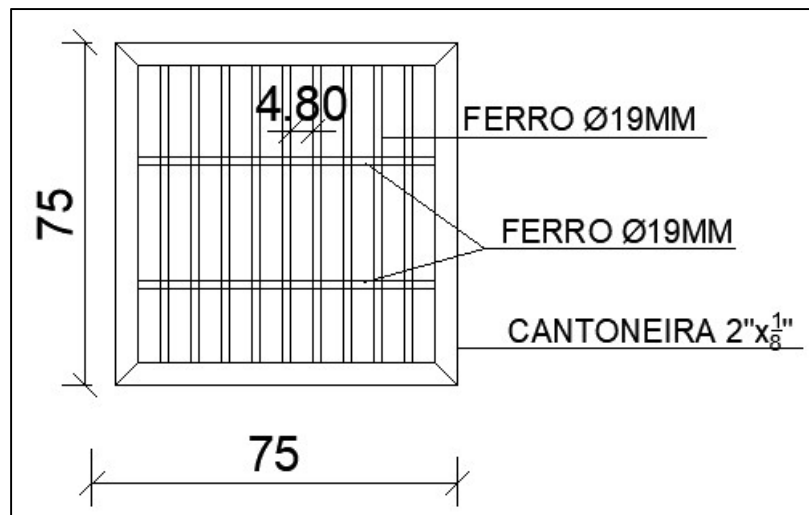
Figura 1: Detalhamento Grelha.
