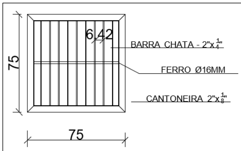
Figura 2 Detalhamento Grelha - Ferro chato
