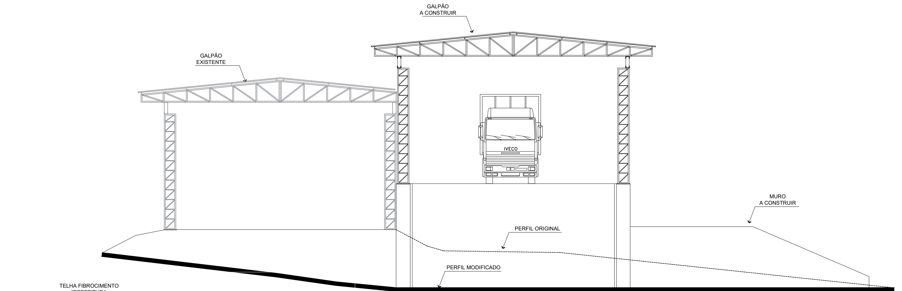
VISTA FRONTAL ESC.: 1:100
