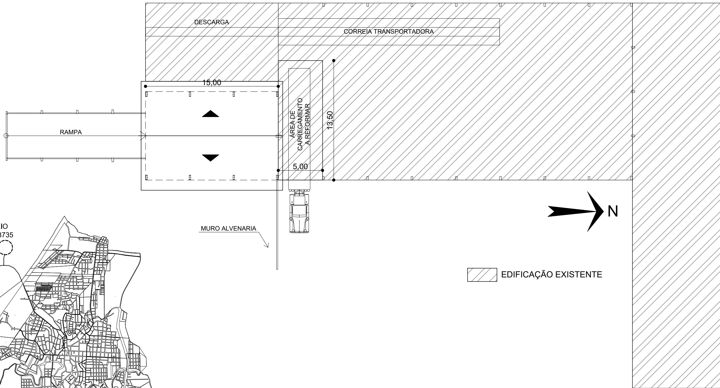
PLANTA DE LOCALIZAÇÃO ESC.: 1:250
