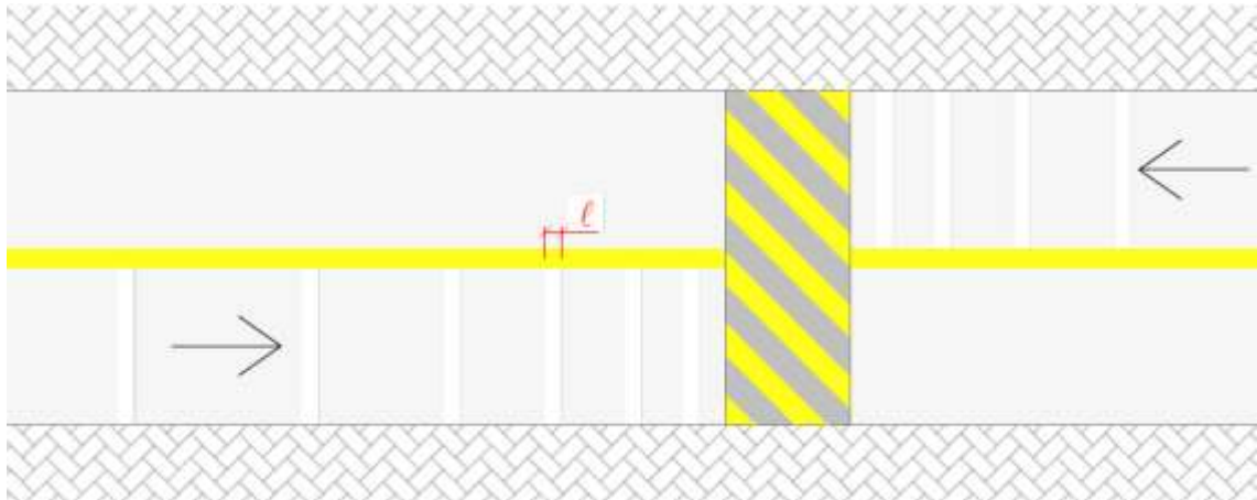
Figura 9 Linha de estímulo a redução de velocidade
