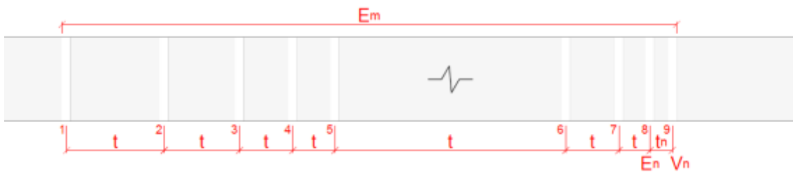
Figura 9 Linha de estímulo a redução de velocidade
