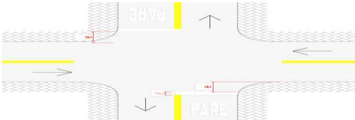
Figura 8 Linha de retenção branca
