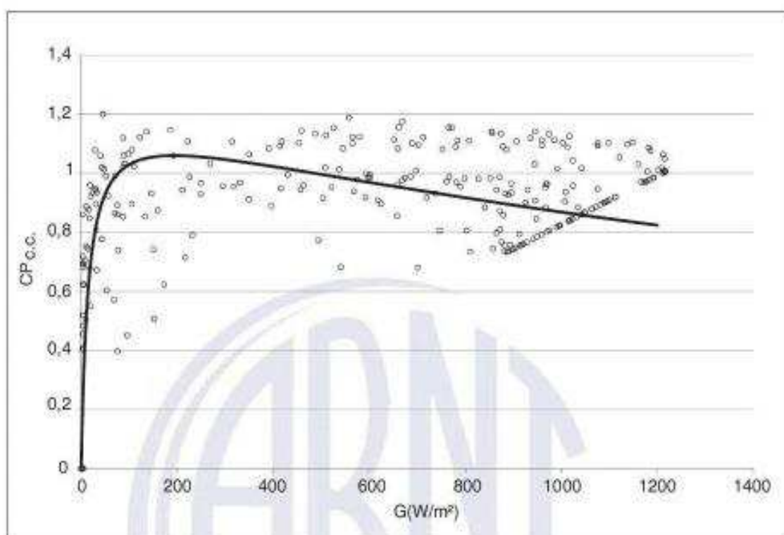
Figura F.2 – Curva do comportamento médio da nuvem de pontos de CP_{c.c.}
