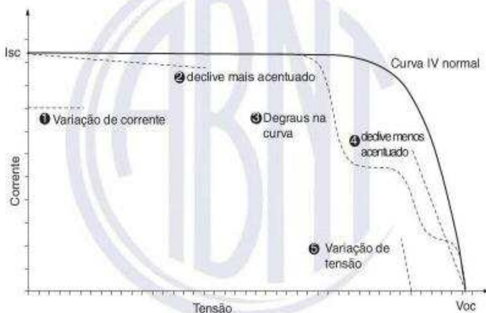
Figura C.1 – Variações na forma da curva IV
