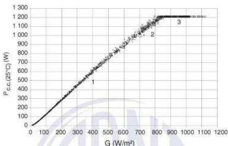
Figura D.1 – Exemplo de curva P_{c.c.(25^{\circ}C)} \times G_C de um arranjo fotovoltaico de 1,5 kWp
