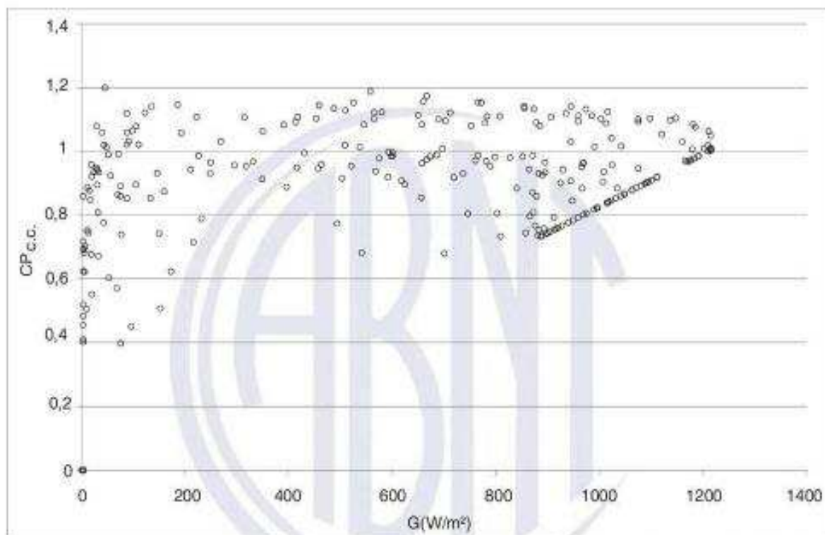
Figura F.1 – Exemplo de nuvem de pontos de CP_{c.c.} para um sistema real
