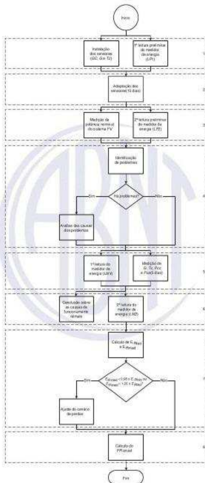
Figura 3 – Fluxograma do procedimento de avaliação de desempenho tipo 2
