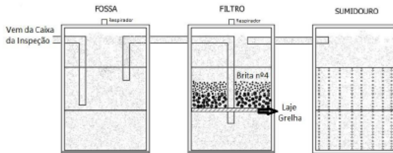
Figura 01 – Sistema de Esgoto
