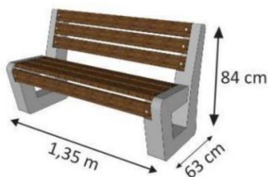
Figura 3. Banco com encosto com estrutura em concreto
