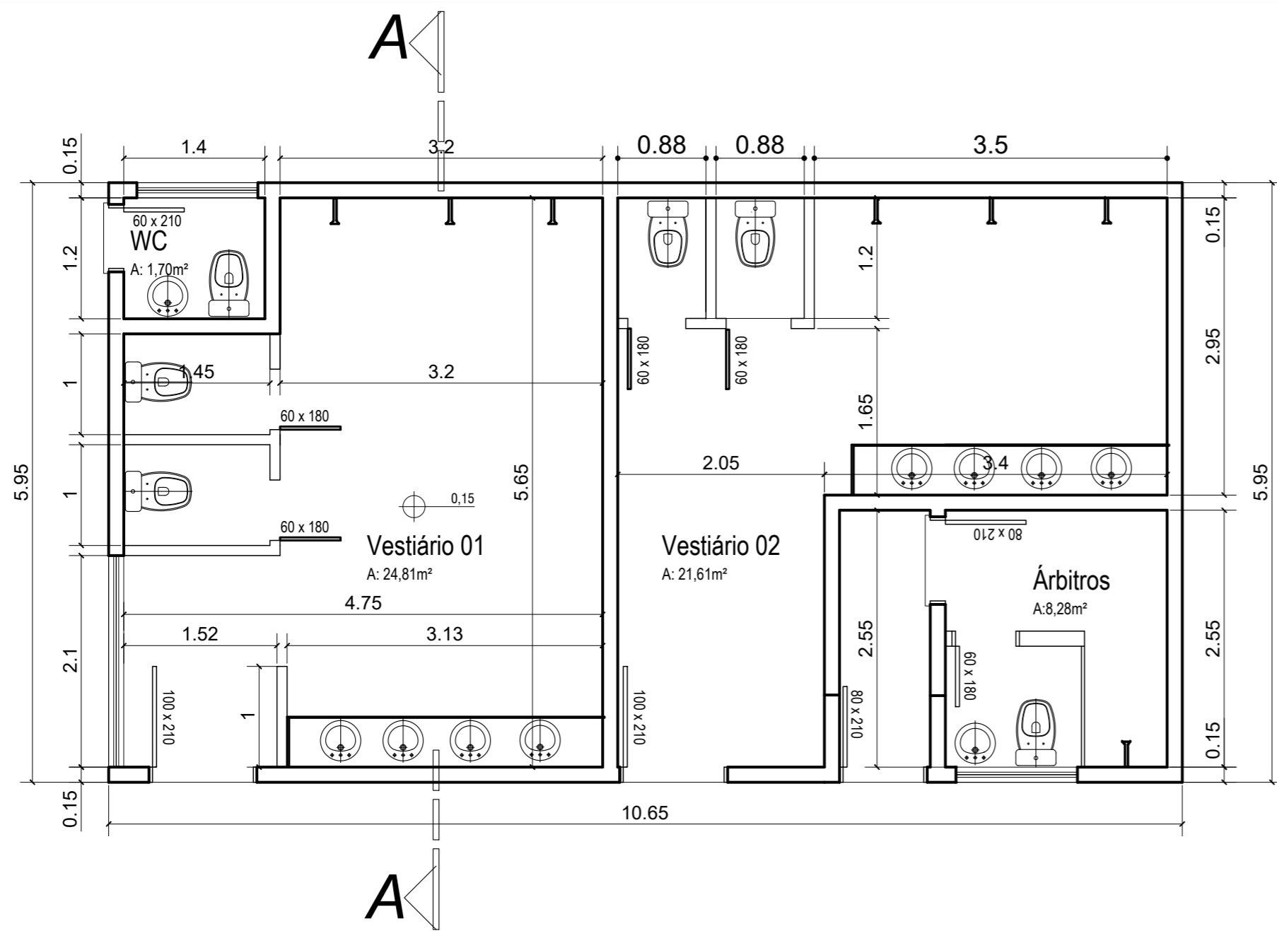
PLANTA BAIXA ESCALA 1/250
