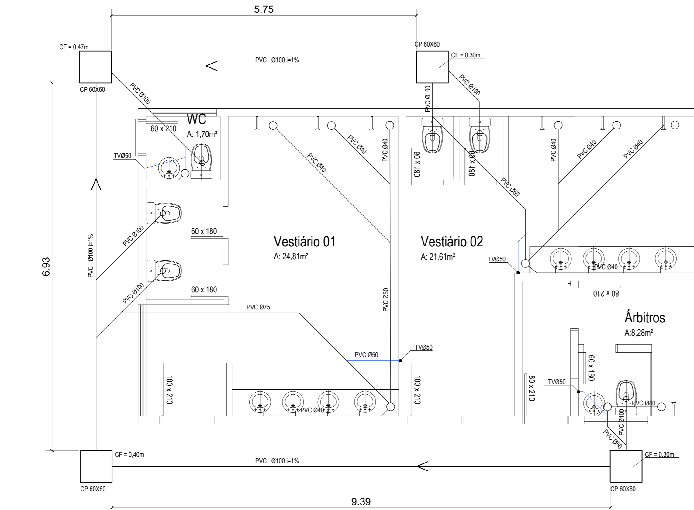
PLANTA BAIXA ESCALA 1/250
