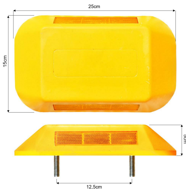
Modelo de tachões bidirecionais para zebrações e canalizações
