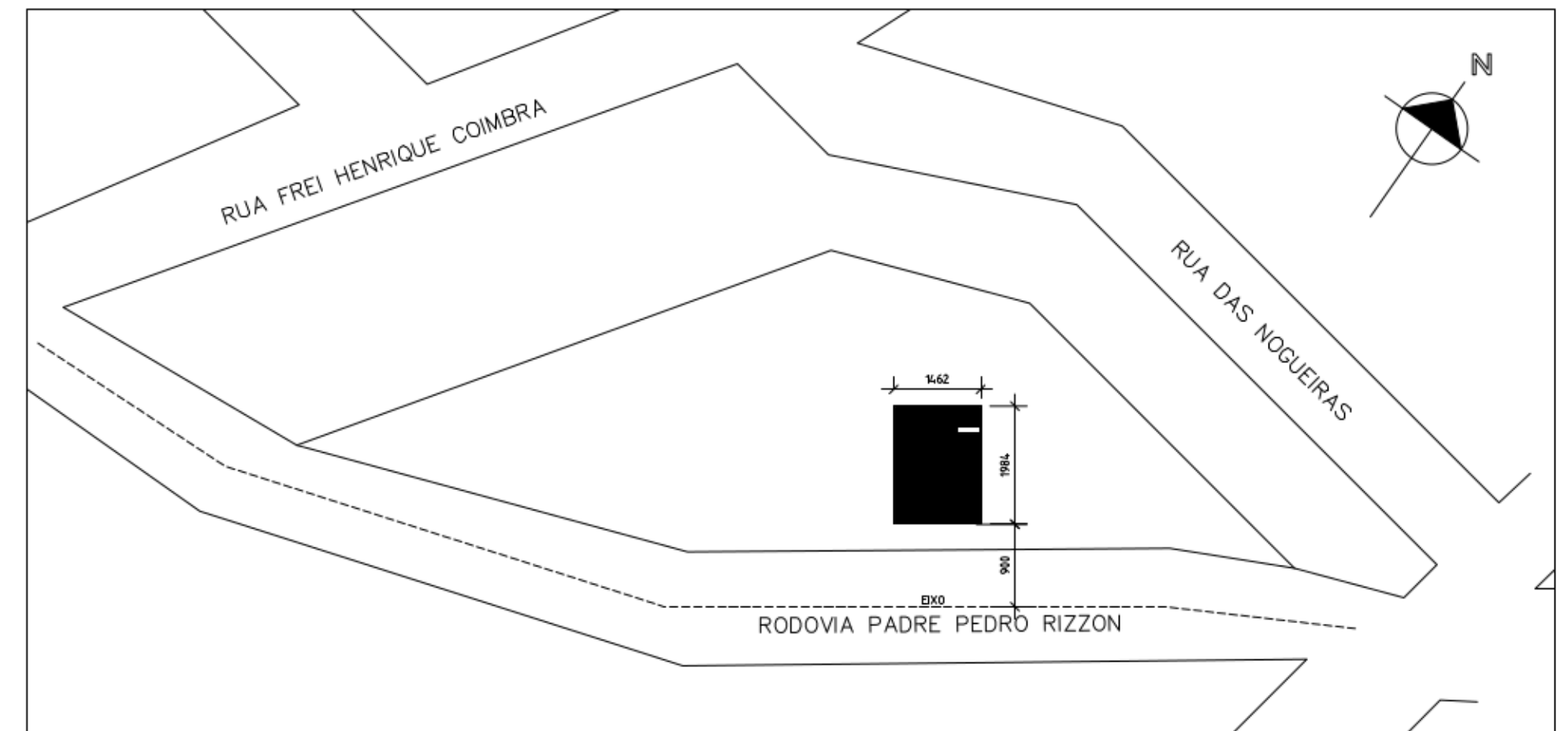
PLANTA DE SITUAÇÃO E LOCALIZAÇÃO Escala 1:1000
