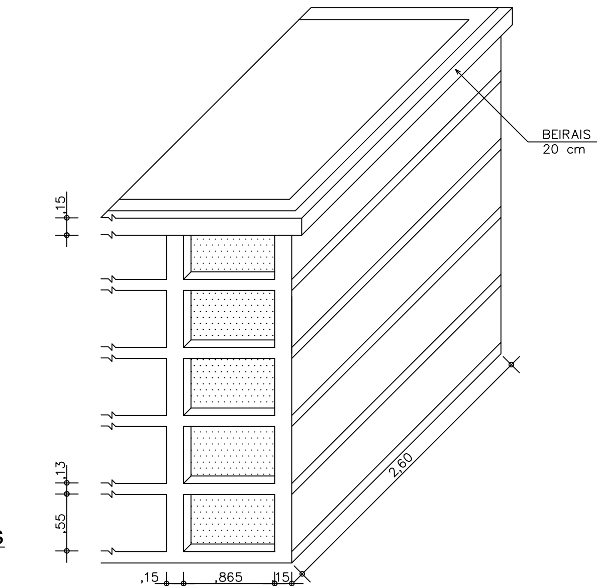
5 Detalhe gavetas S/ Escala
