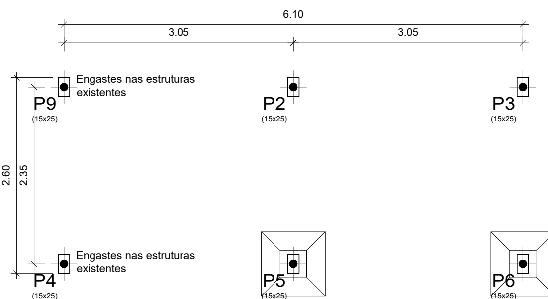
3 Localização Fundações Esc.1/50
