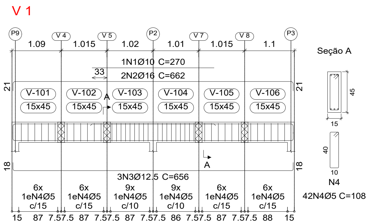
4 Detalhamento Vigas Esc.1/50 Corte 1/25
